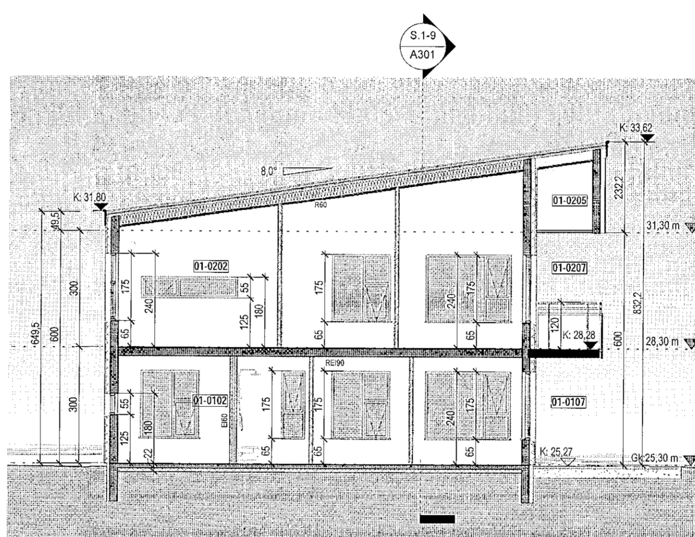
Snið 4 1:100
