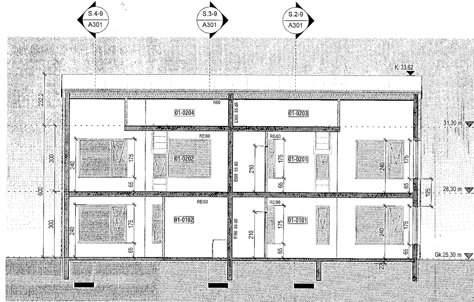
Snið 1 1:100
