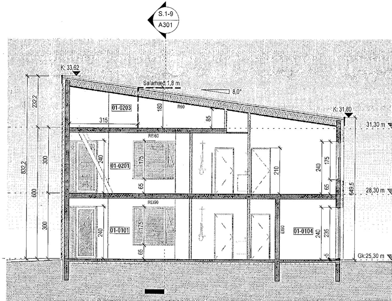
Snið 2 1:100
