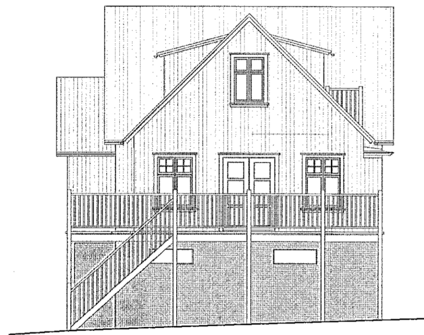
Útlit norður 1:100
