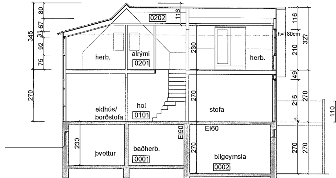
Sneiðing aa 1:100
