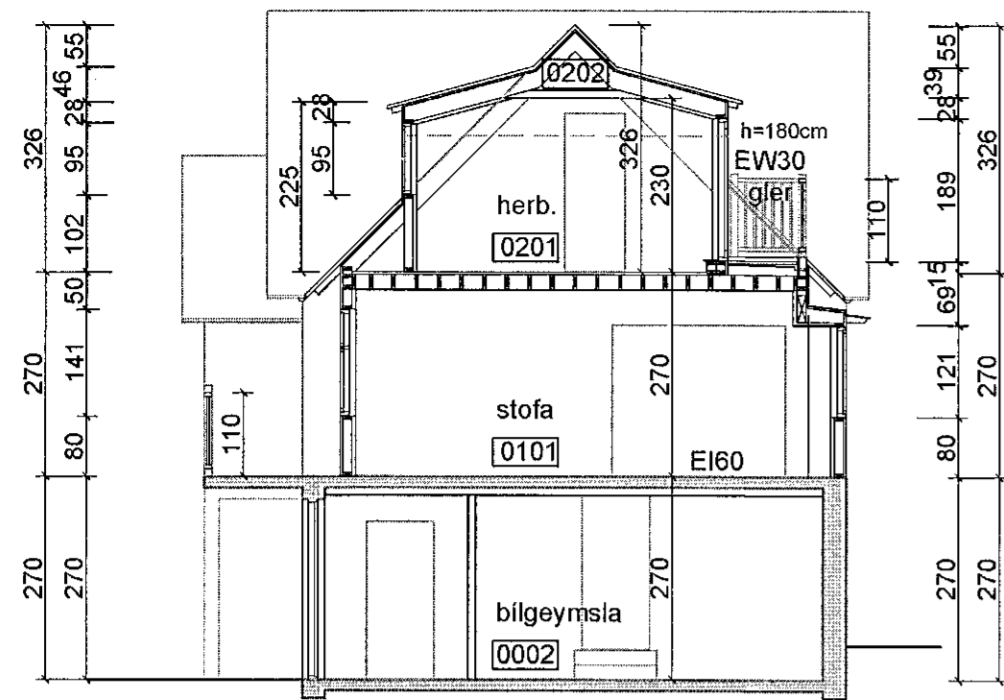
Sneiðing bb 1:100
