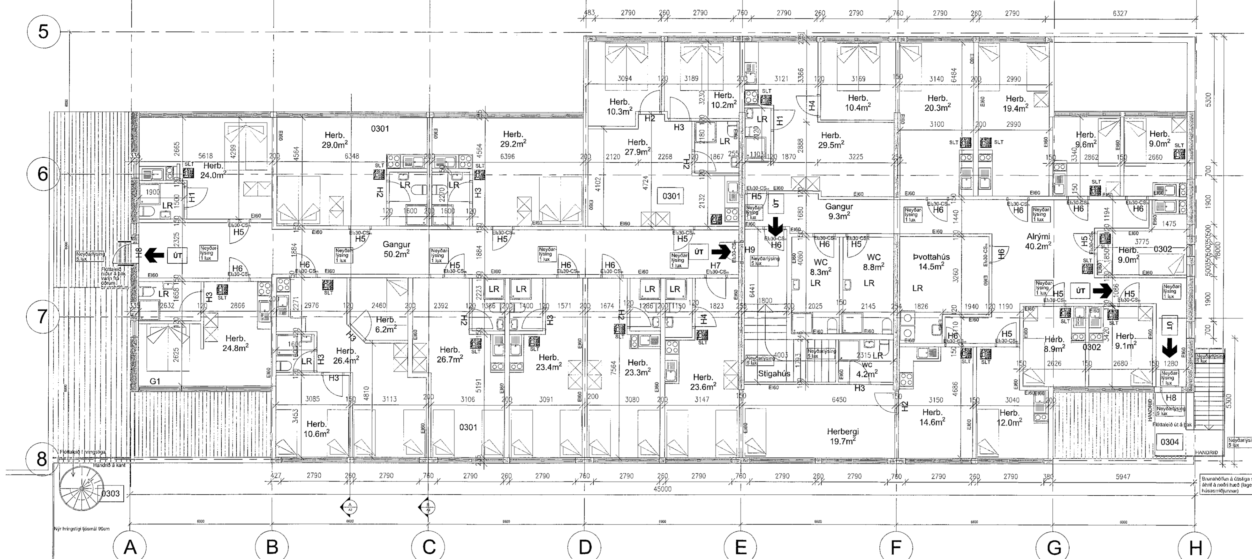
Grunnmynd 3.hæð M 1:100
