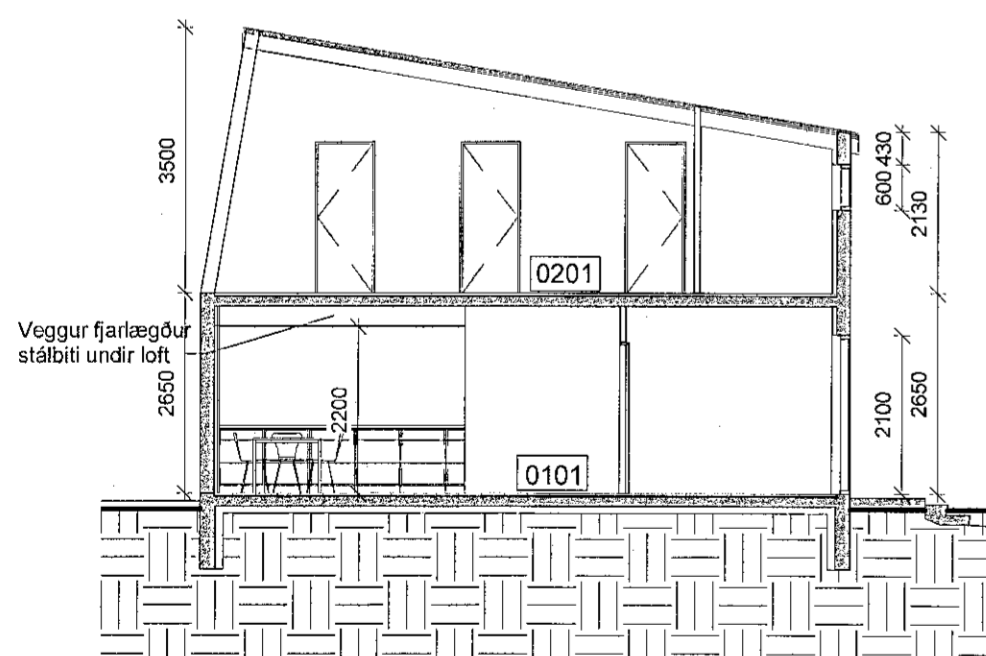
A-A 1 : 100
