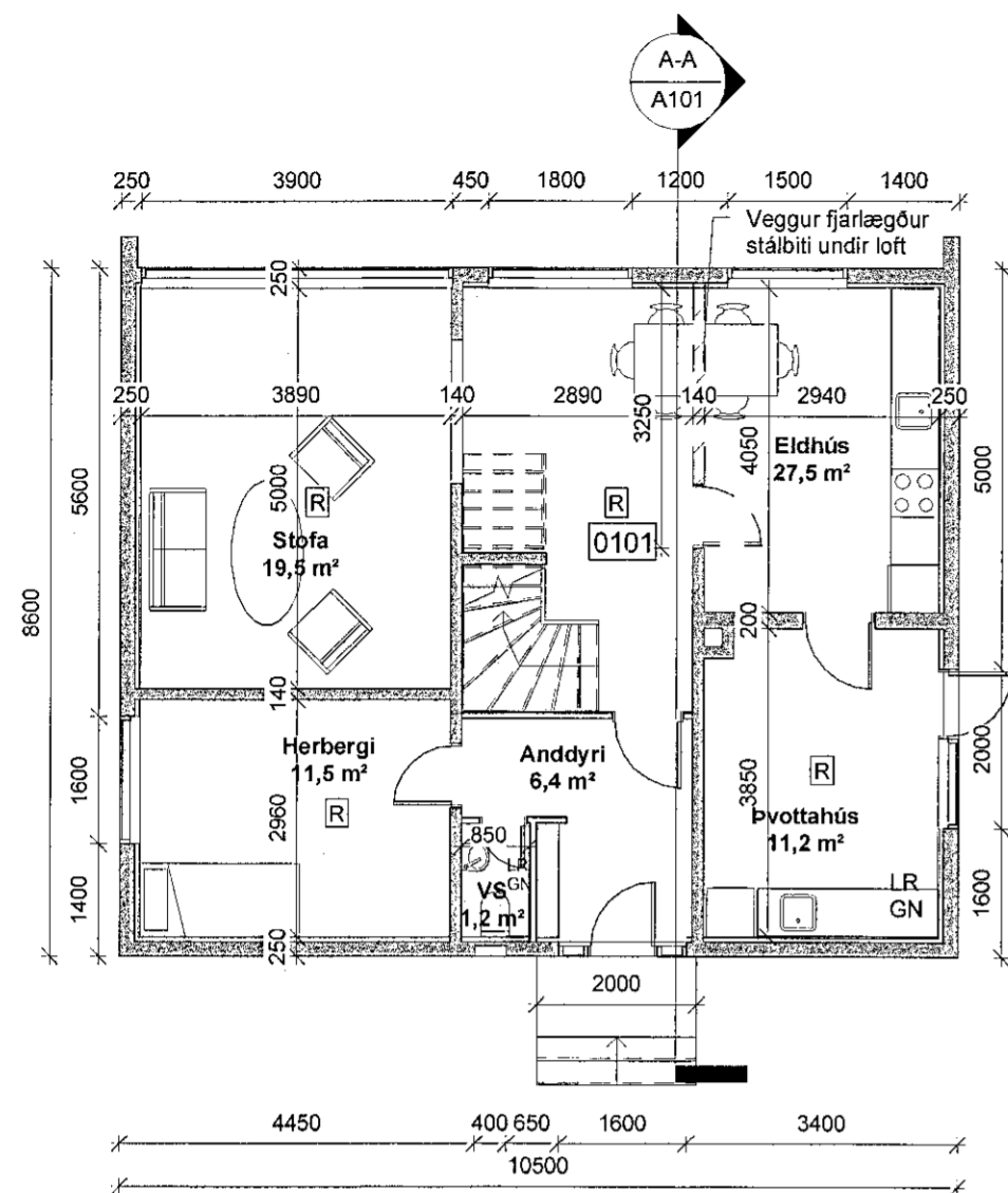
GRUNNMYND 1.HÆÐAR 1 : 100
