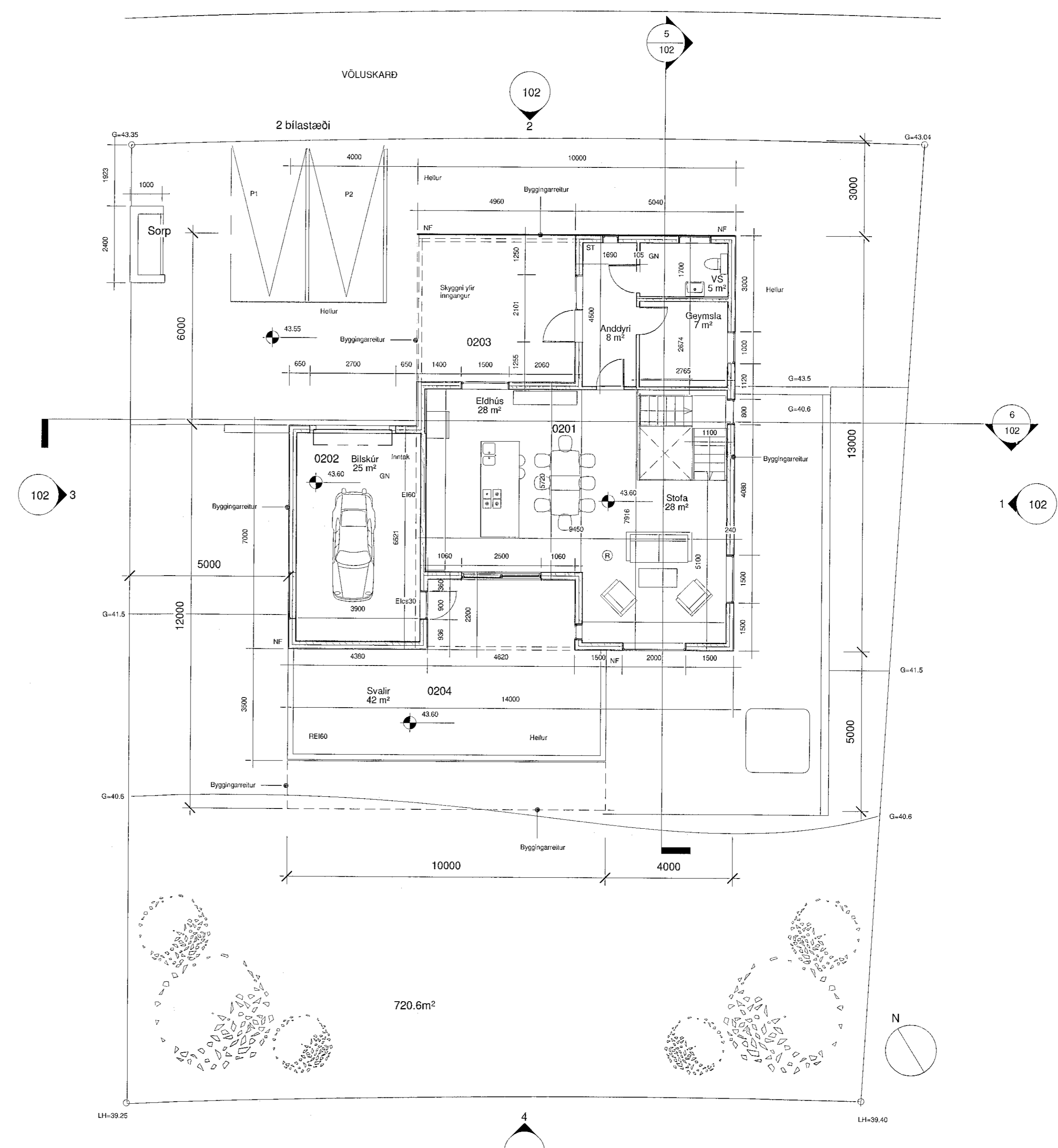
1 2.Hæð 1:100
