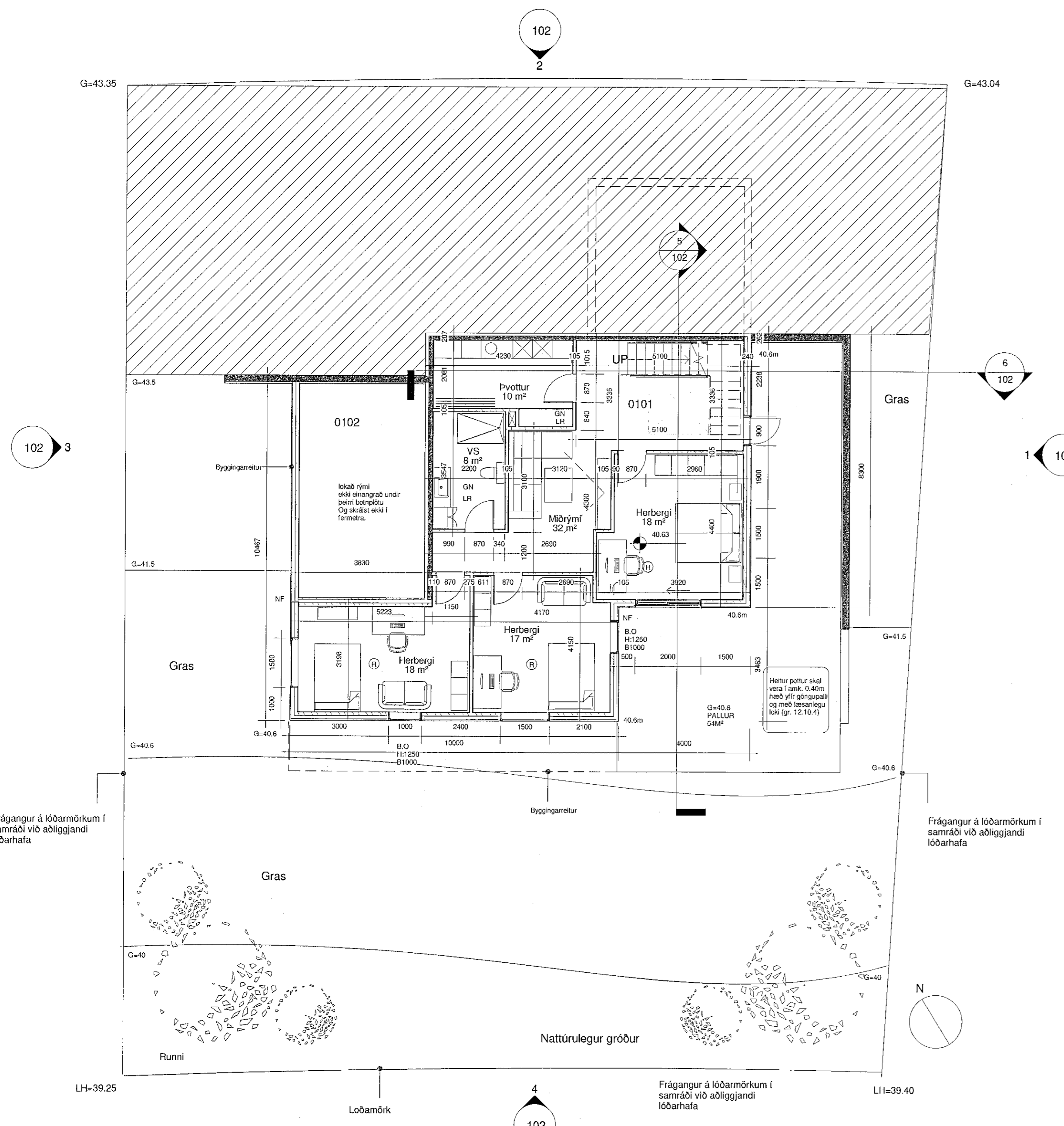
2 1.Hæð 1:100
