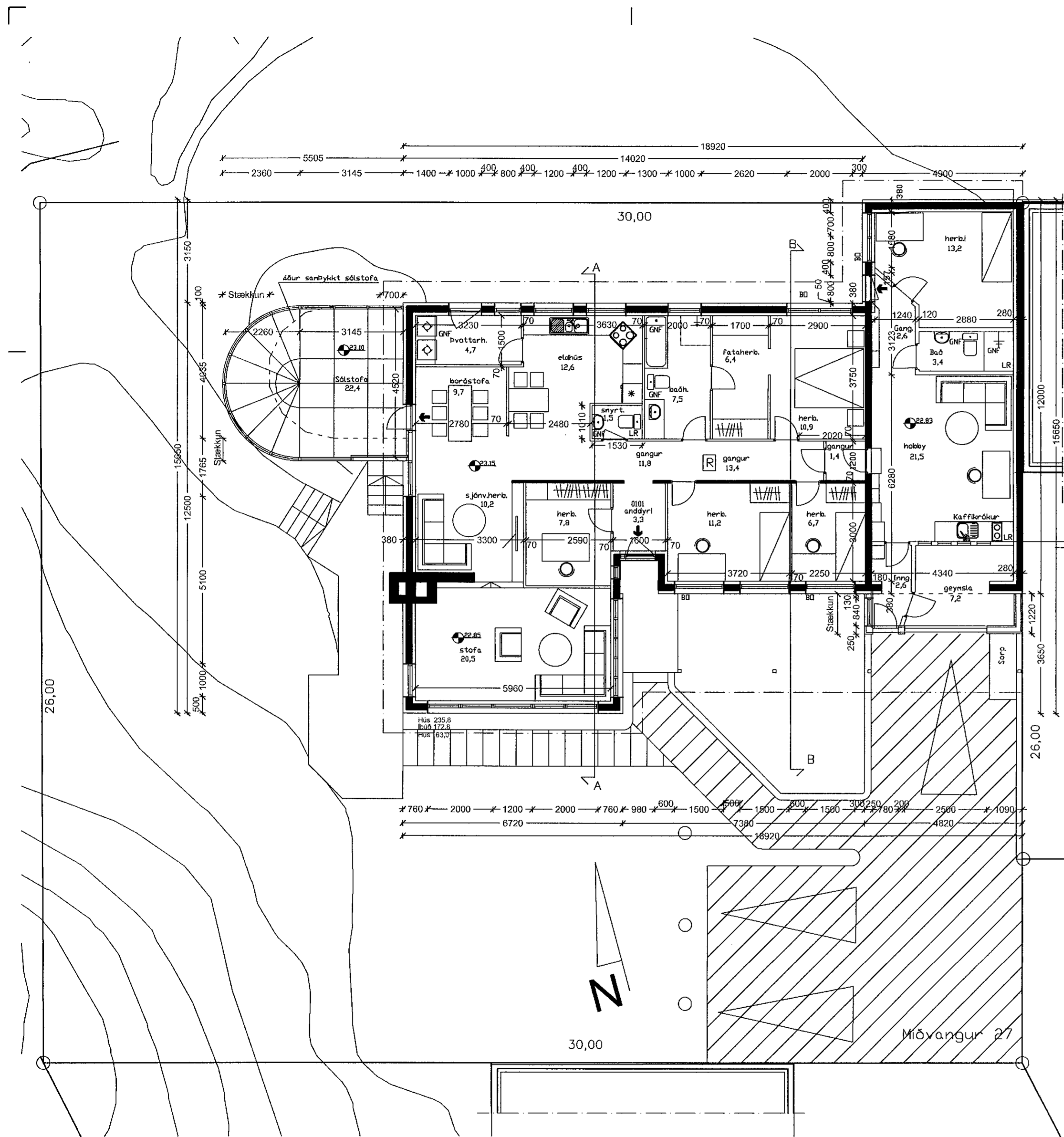
Grunnmynd 1 : 100
