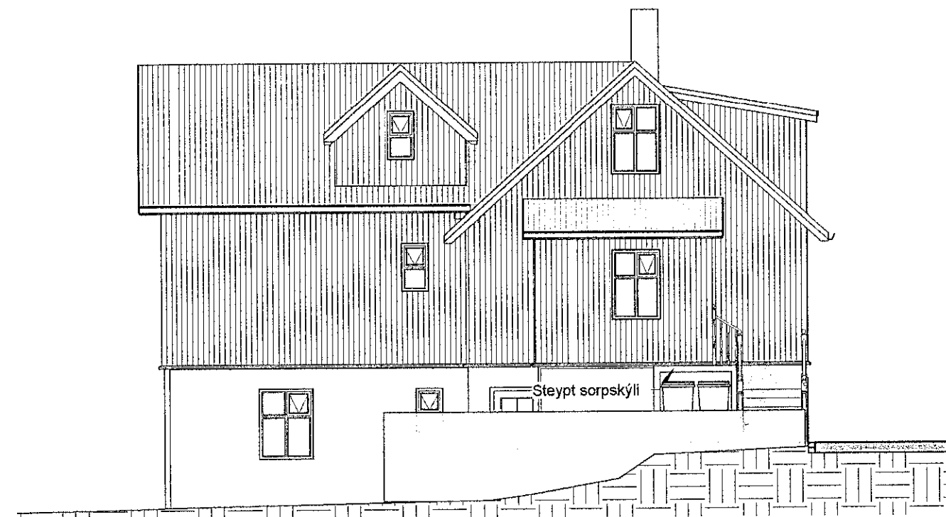
4 NORÐ- AUSTURHLIÐ 1 : 100
