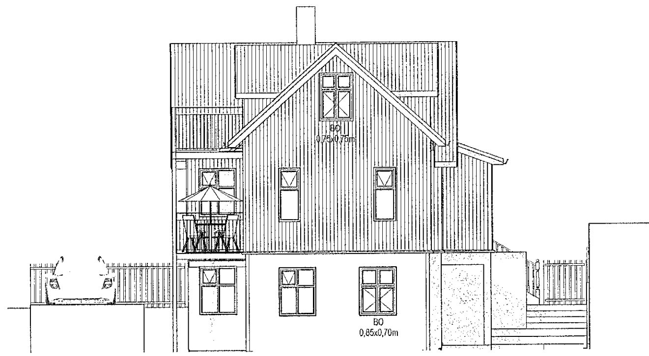
2 SUÐ-AUSTURHLIÐ 1 : 100
