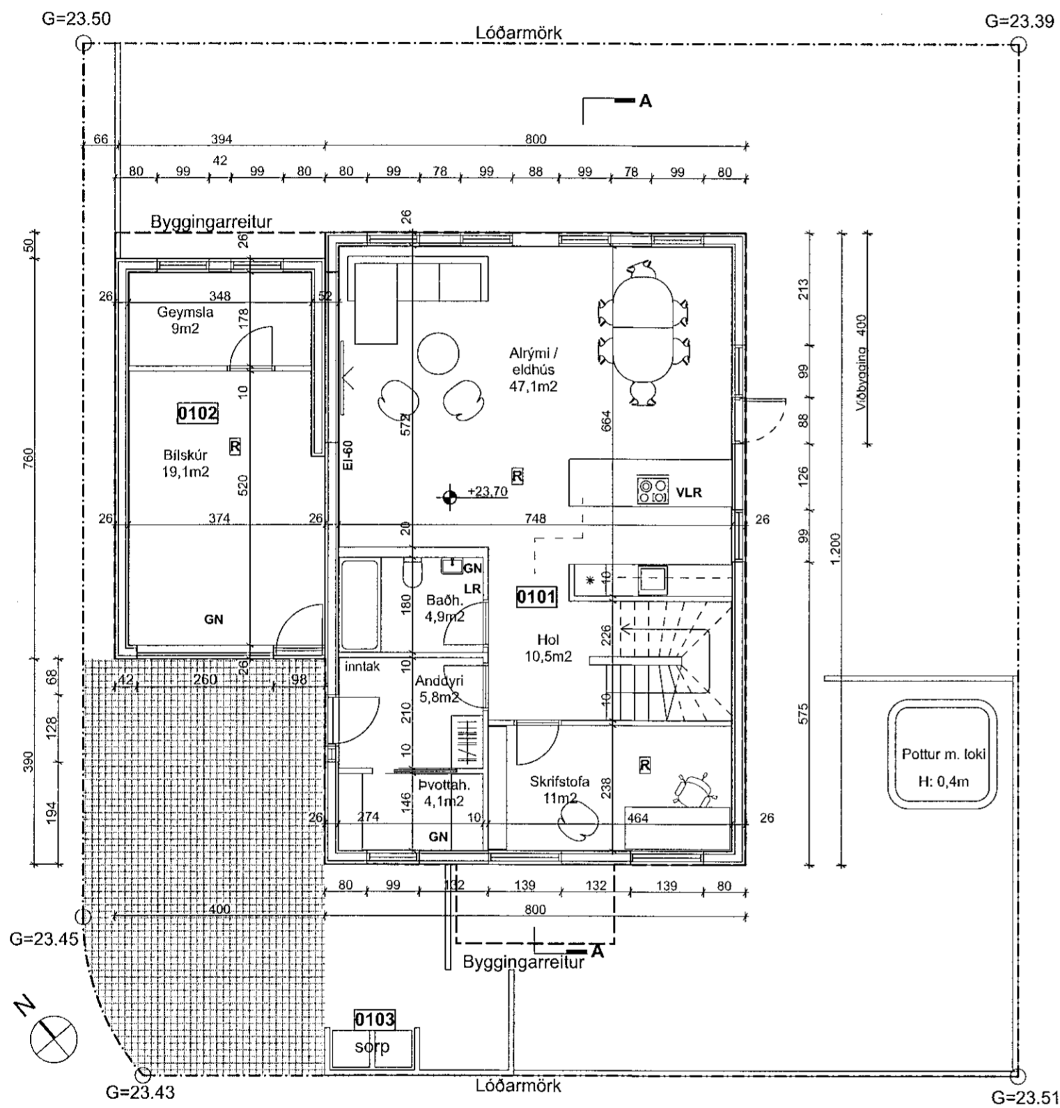
1.hæð 1:100
