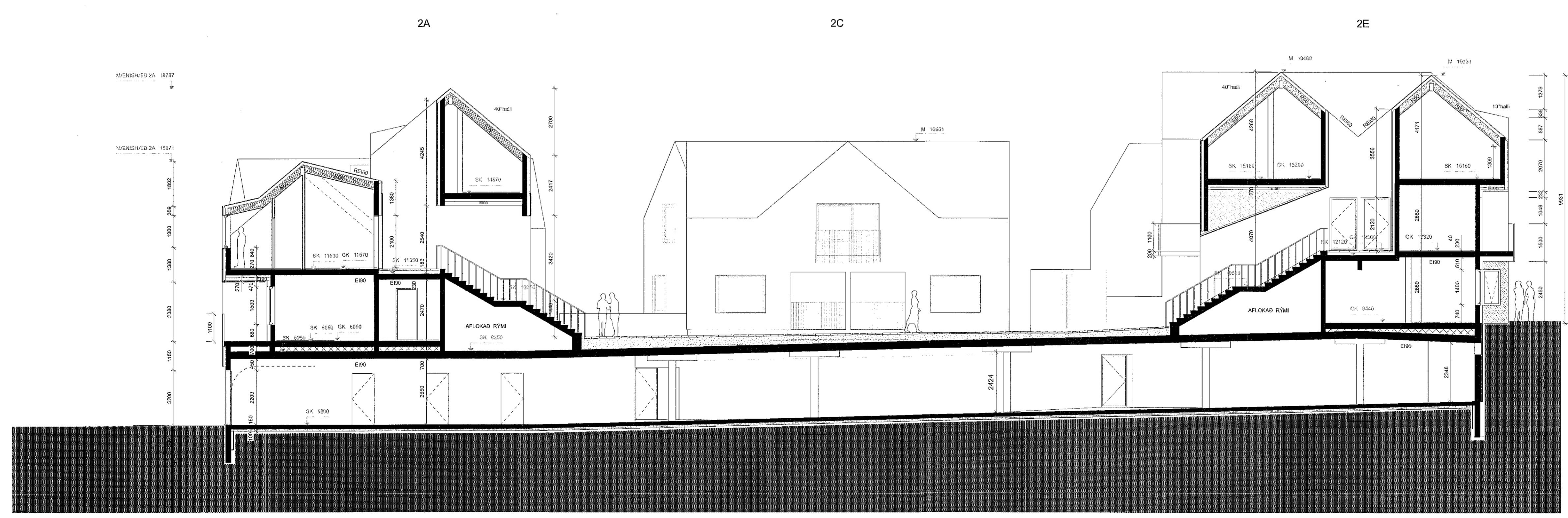
2 SNEIÐING B-B Skali: 1:100
