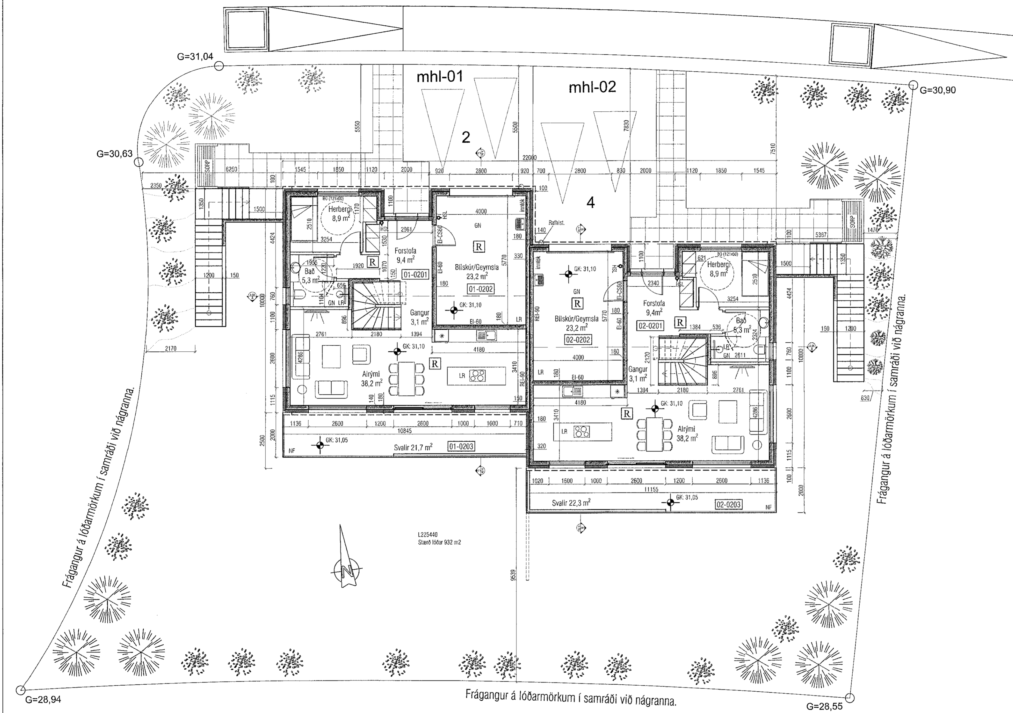
GRUNNMYND 1. HÆÐ 1:100
