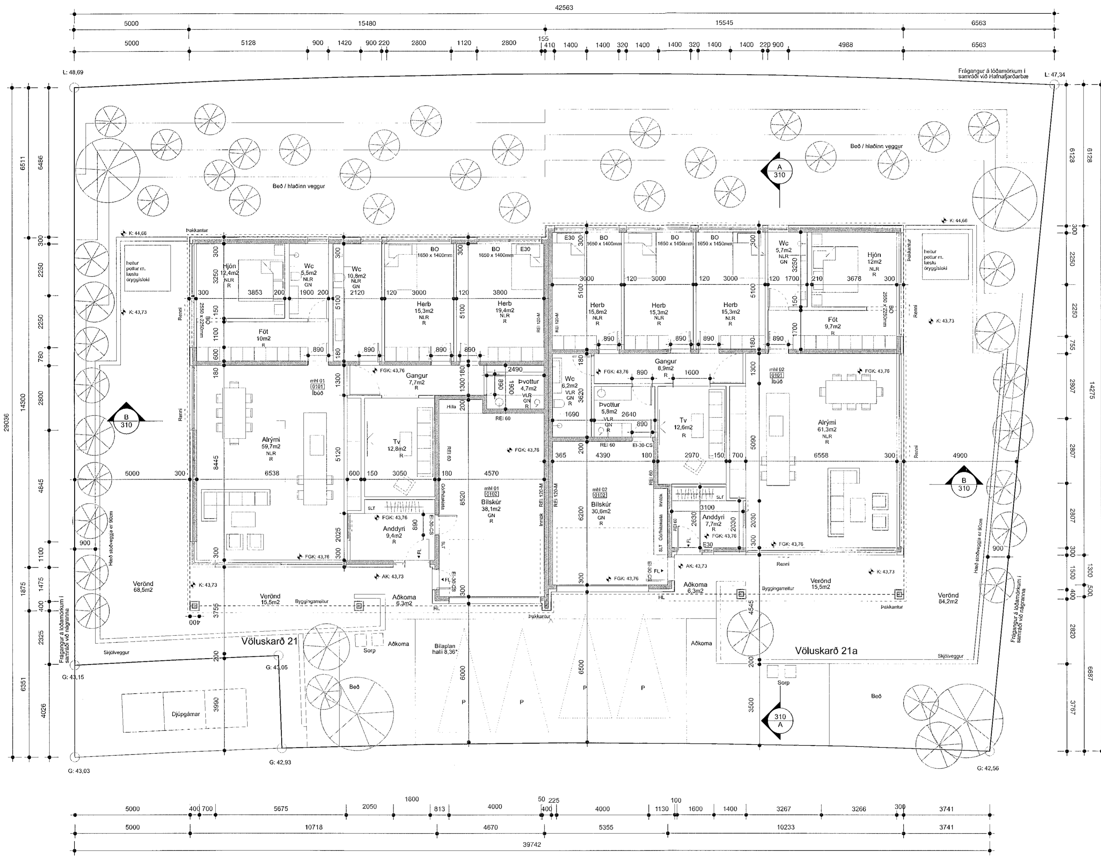
Grunnmynd mkv: 1:100
