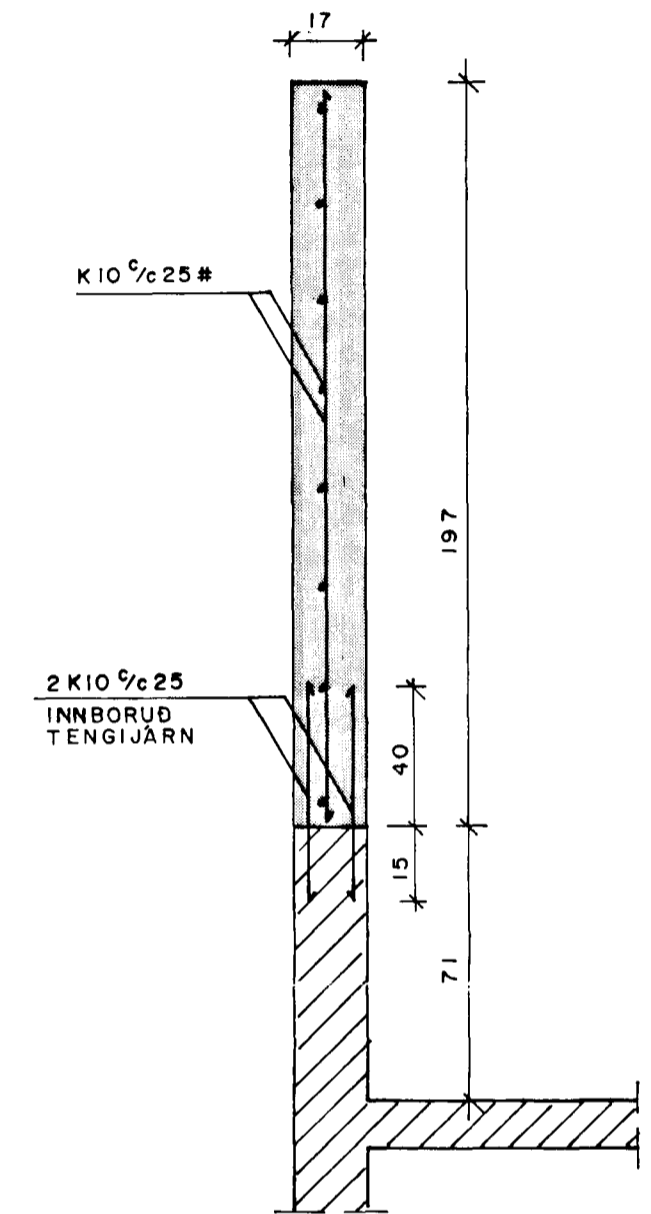
SNID B-B 1:20
