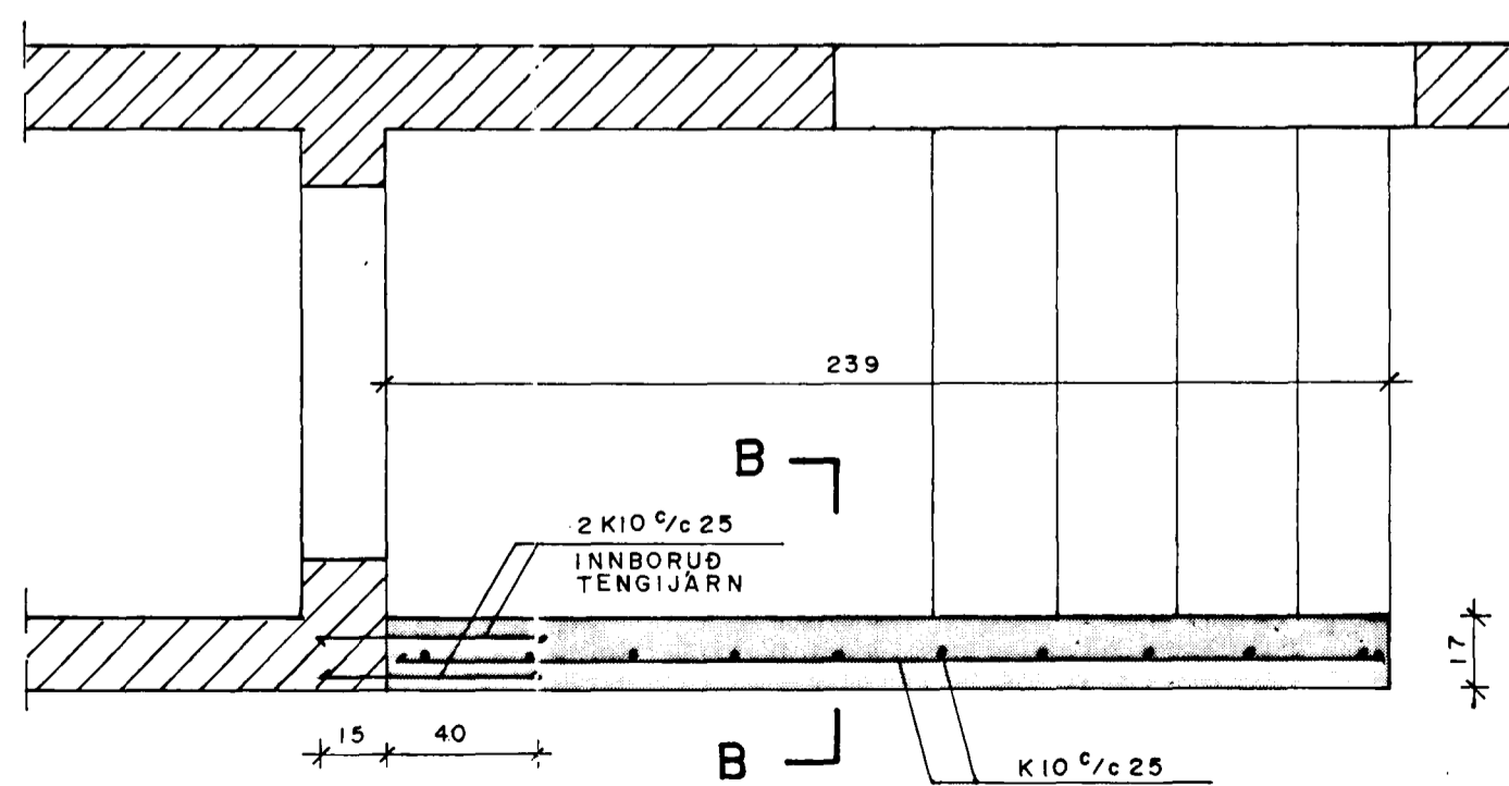
SNID A-A 1:20
