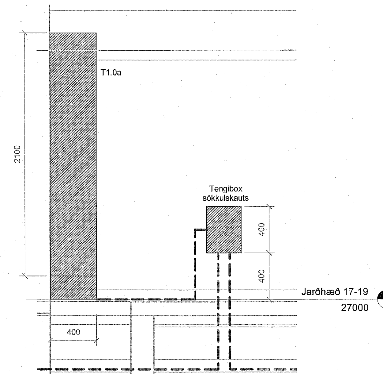
DC Snið DC xx_3_13_61 1 : 20
