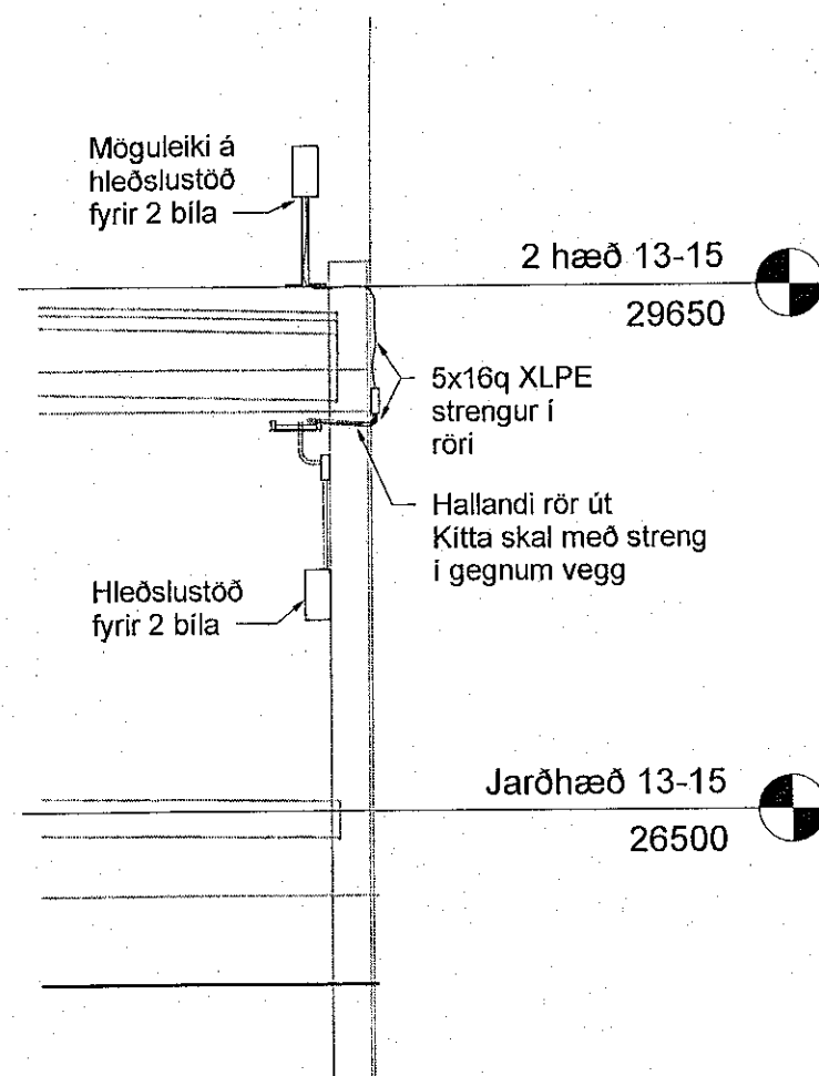
EA Snið EA 00_3_14_04 1:50
