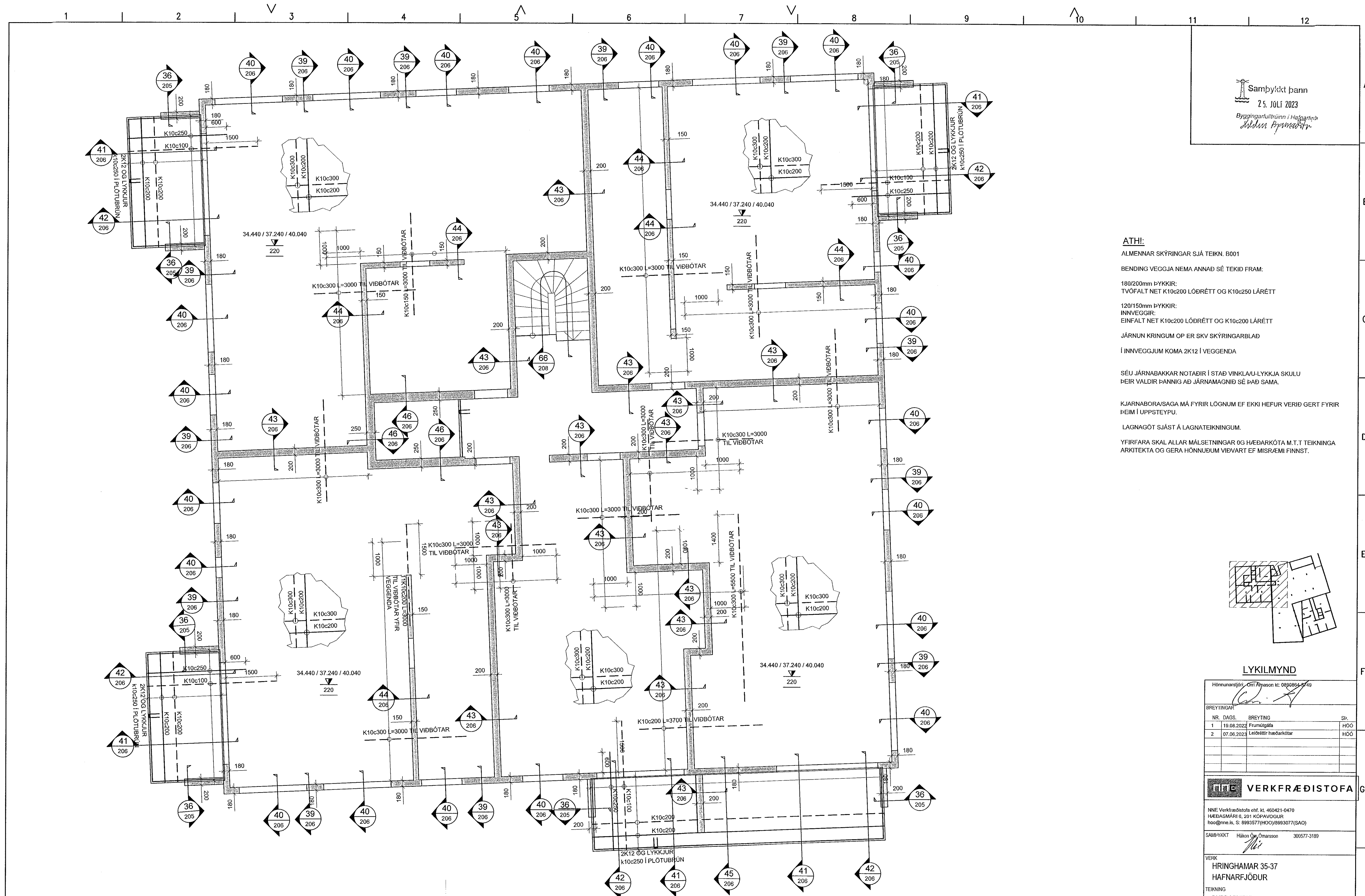
VEGGIR OG LOFTAPLATA 2-4. HÆÐAR, GRUNNMYND MKV. 3
