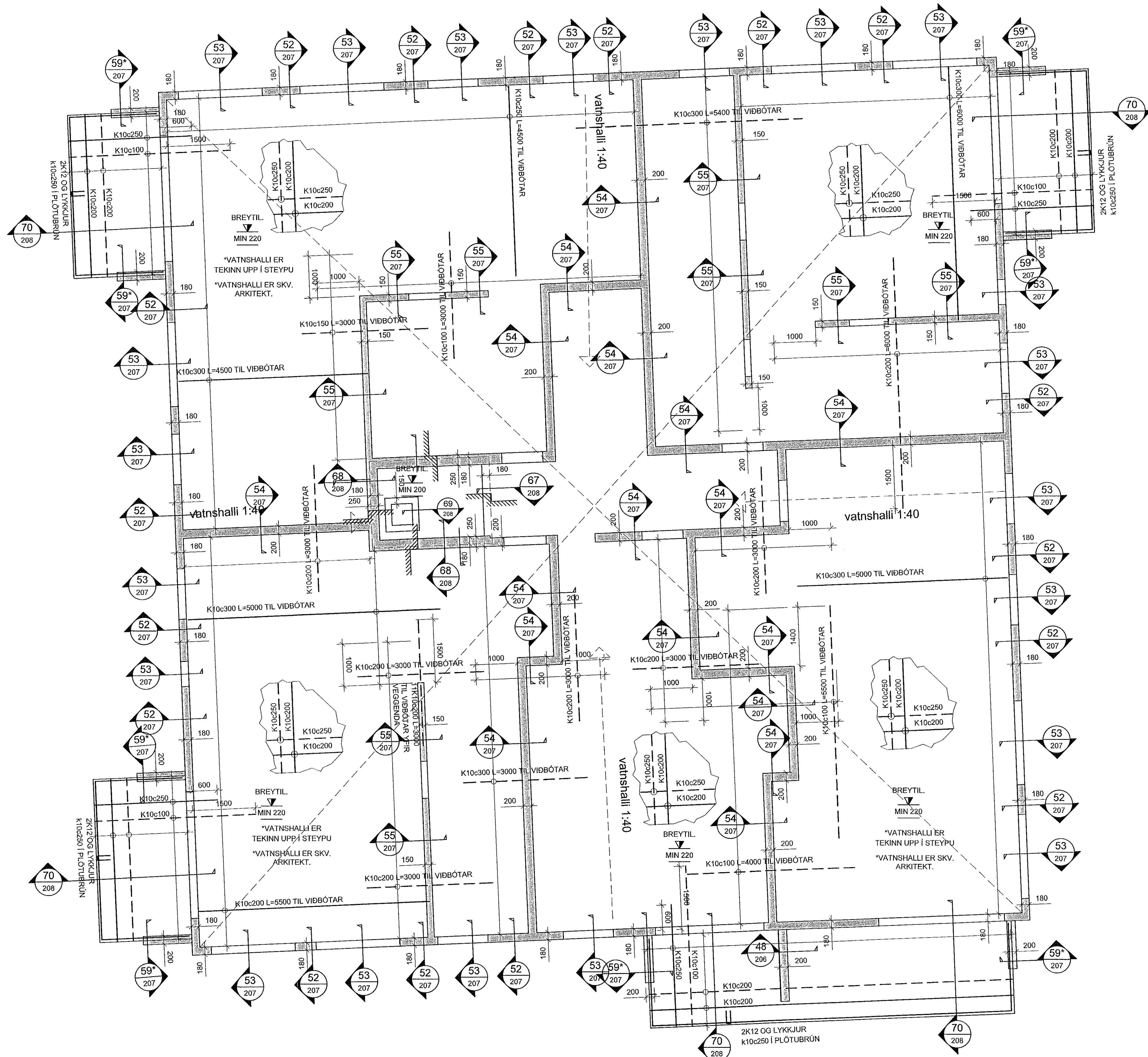
VEGGIR OG LOFTAPLATA 5.HÆÐAR, GRUNNMYND MKV. 3
