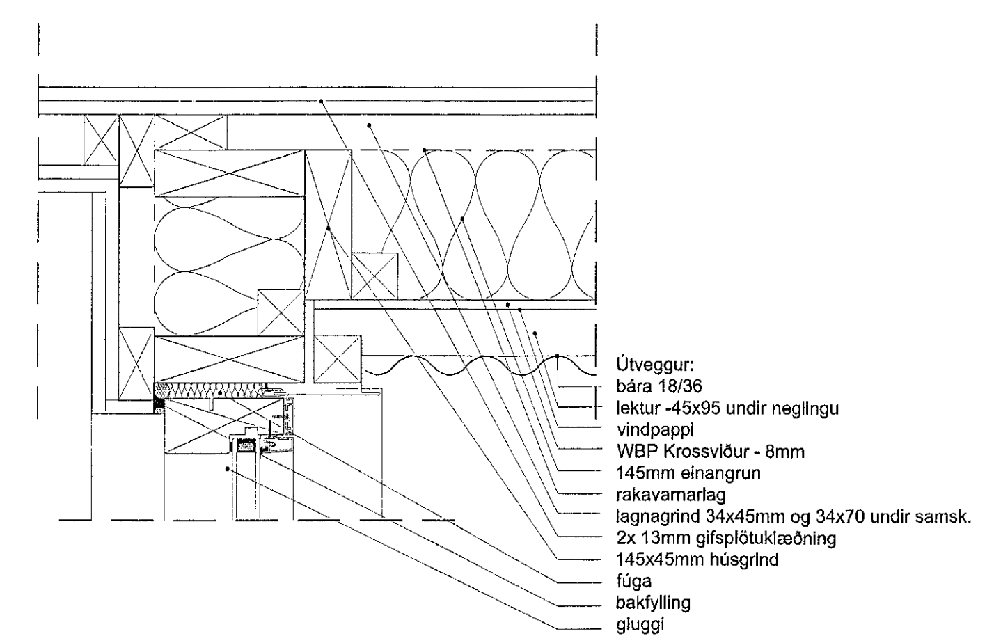
D.04 Lárétt deili við innhorn svala 2.01-01
