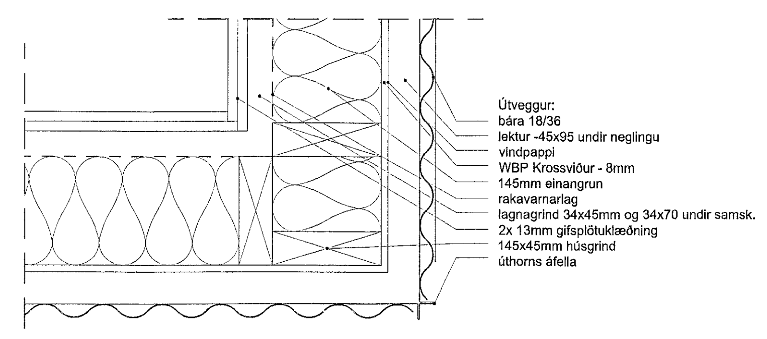
D.05 Lárétt deili við úthorn 2.01-01
