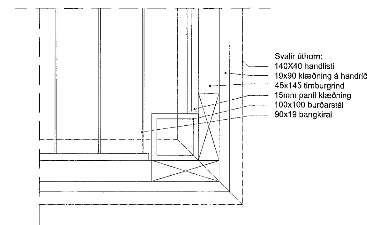
D.03 Lárétt deili við úthorn svala 2.01-01
