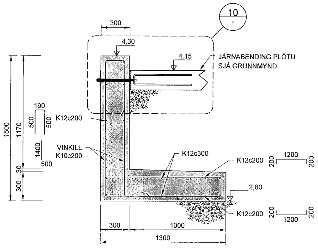
3 SNID 0023 1:20
