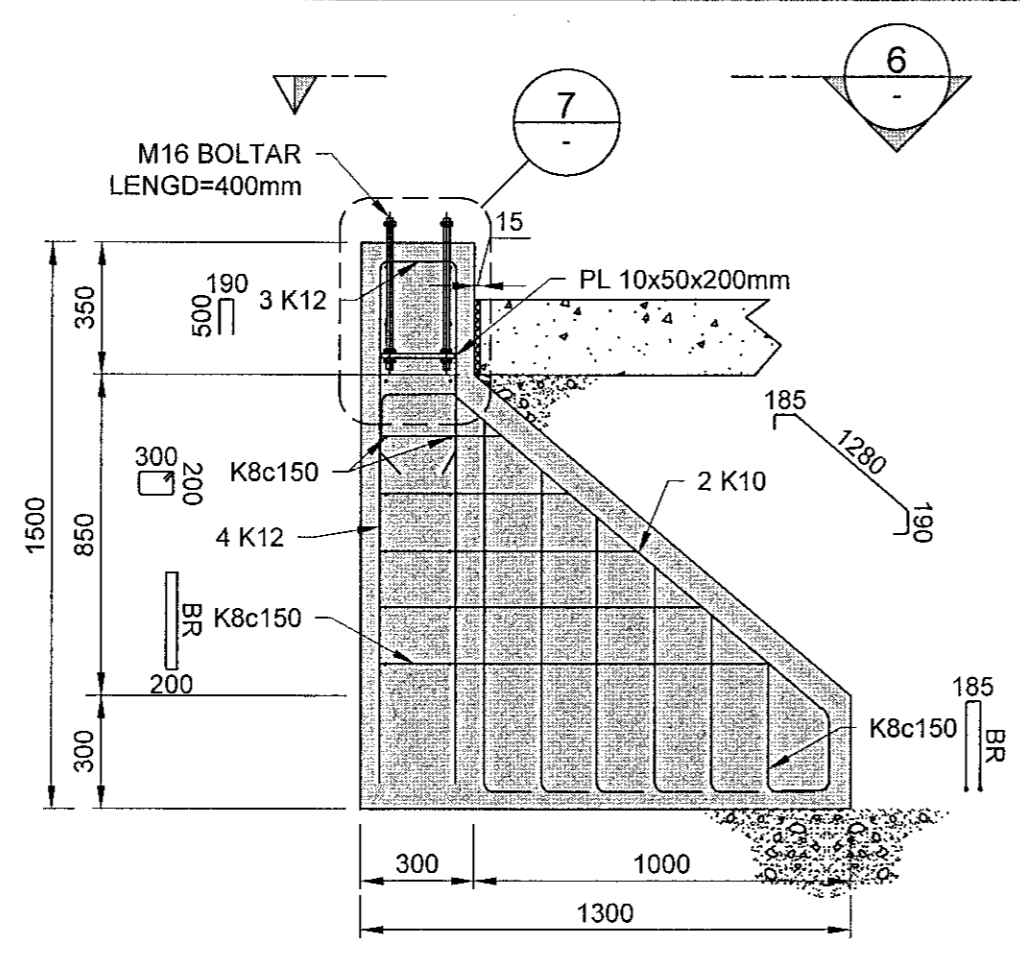
4 SNID 0023 1:20
