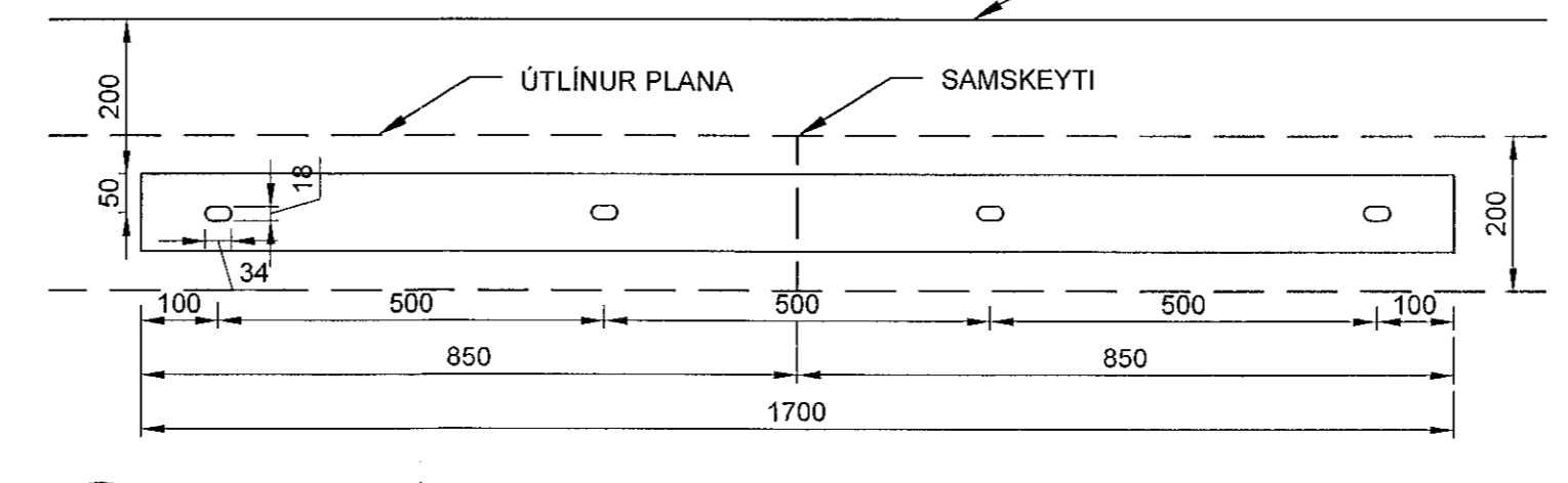
10 DEILI 1:10
