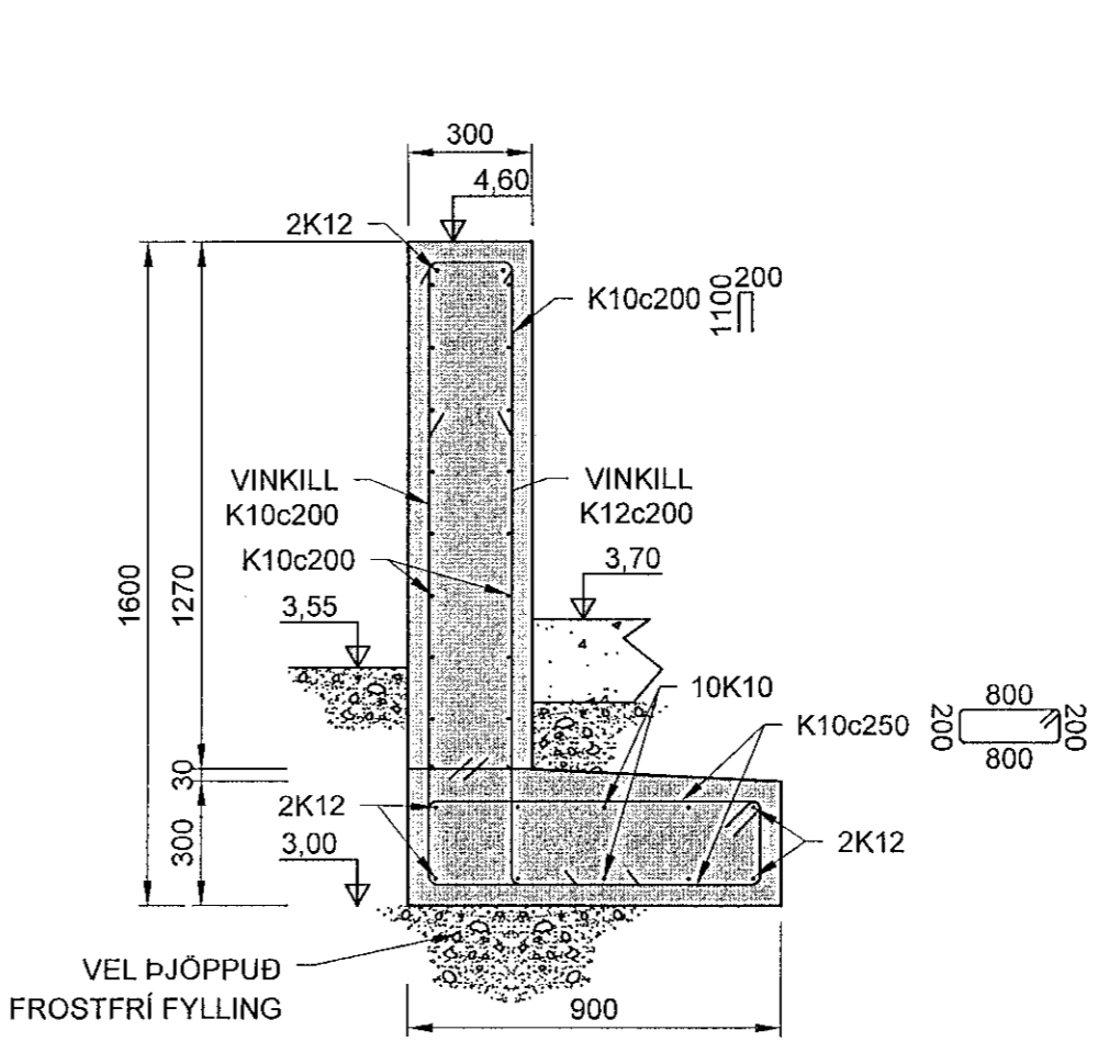
8 SNID 0001 1:20
