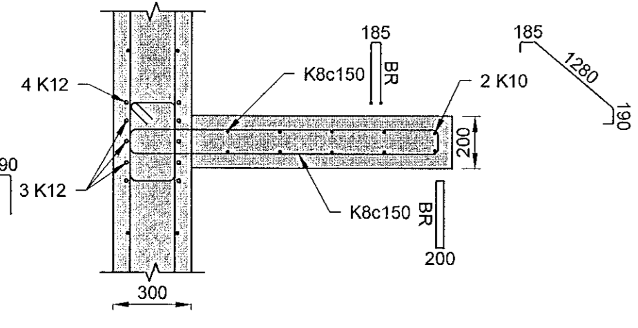
6 SNID 1:20
