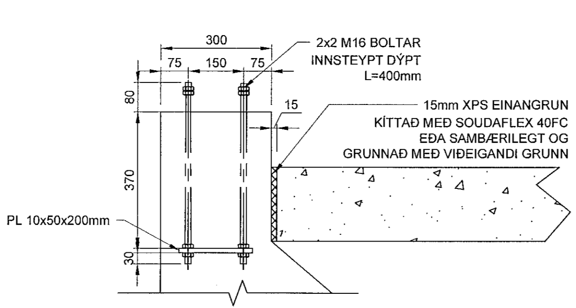
7 DEILI 1:10
