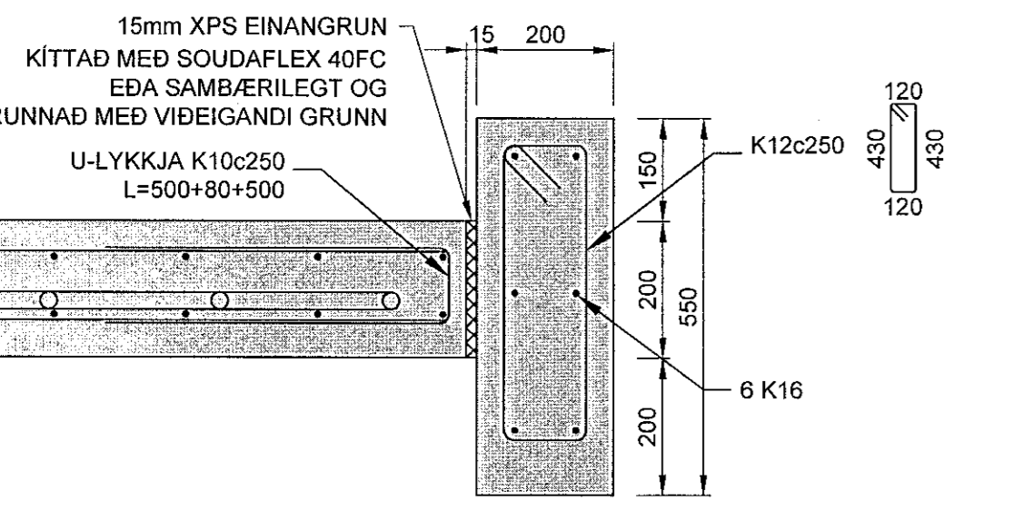
13 DEILI 1:10
