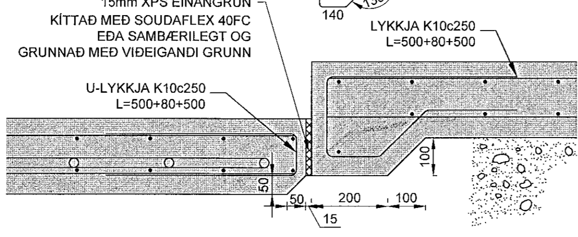
12 SNID 0023 1:10
