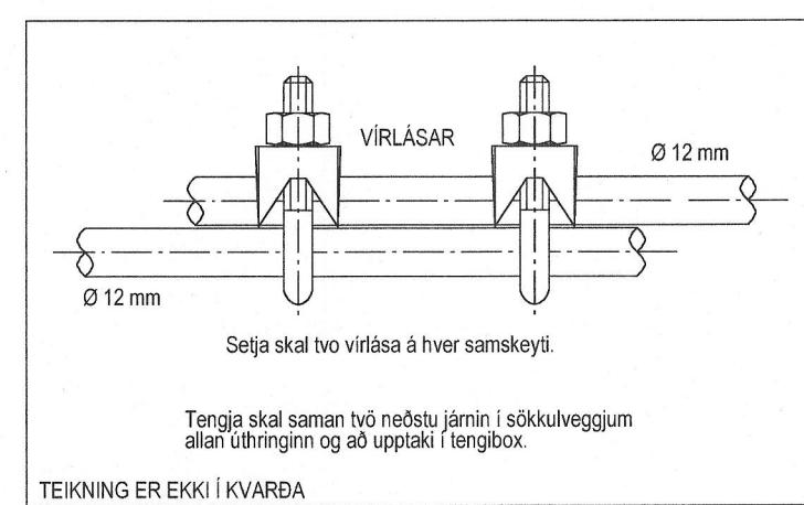
TEIKNING ER EKKI Í KVARÐA SAMTENGING STEYPUSTEINA DEMIGERÐUR FRÁGANGUR
