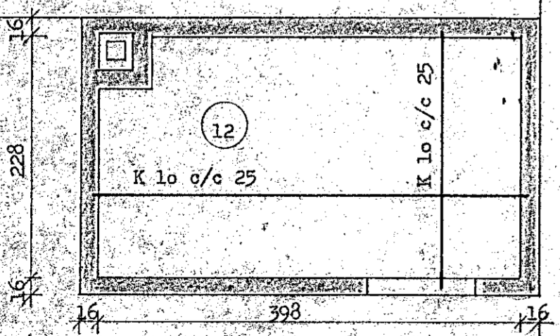
LOFT OG VEGGIR Í HÆÐ 1:50
