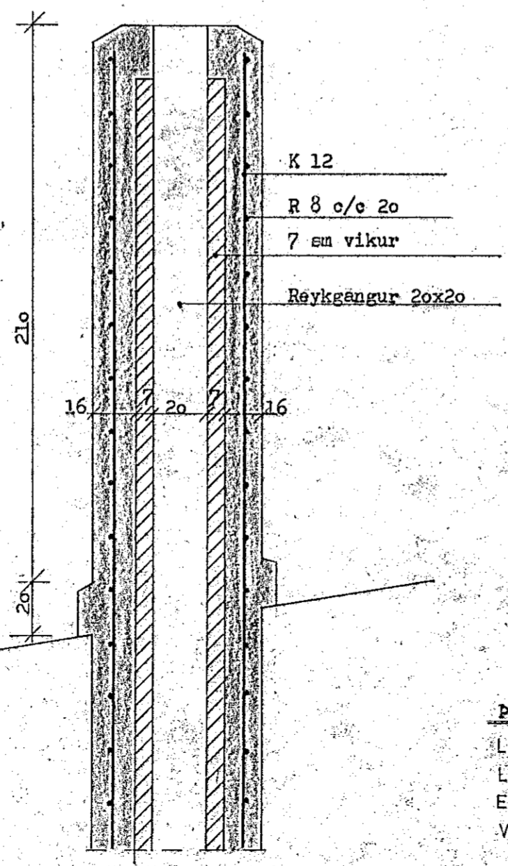
LANGSNID Í REYKHAF 1:20
