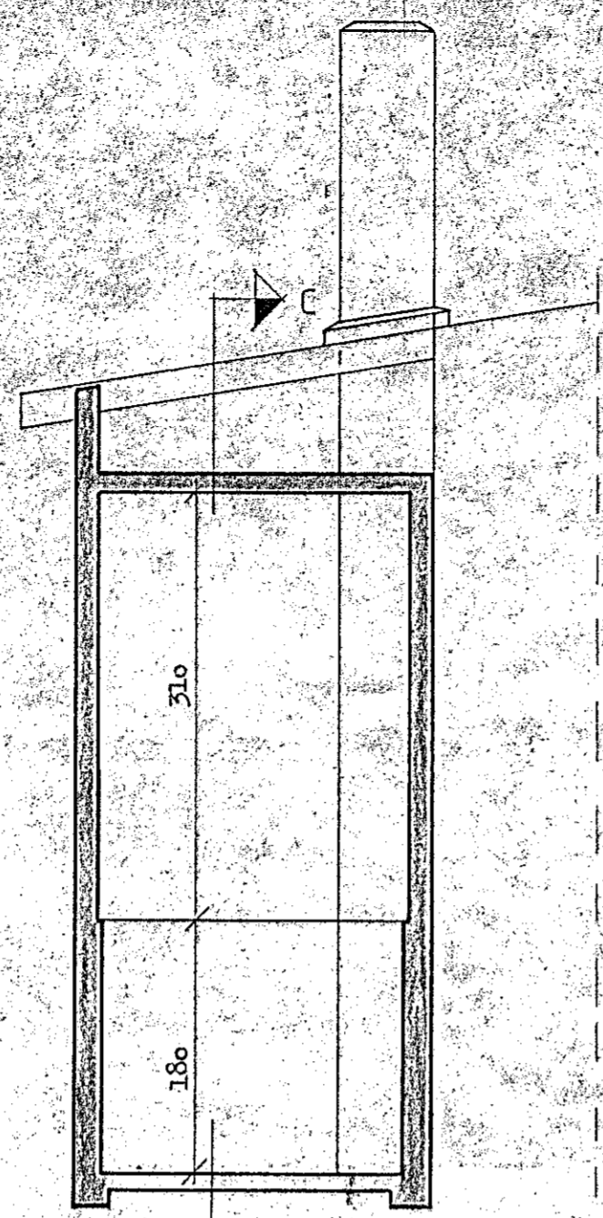
SNID E - E 1:50
