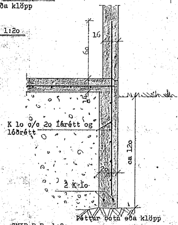
SNID B-B 1:20
