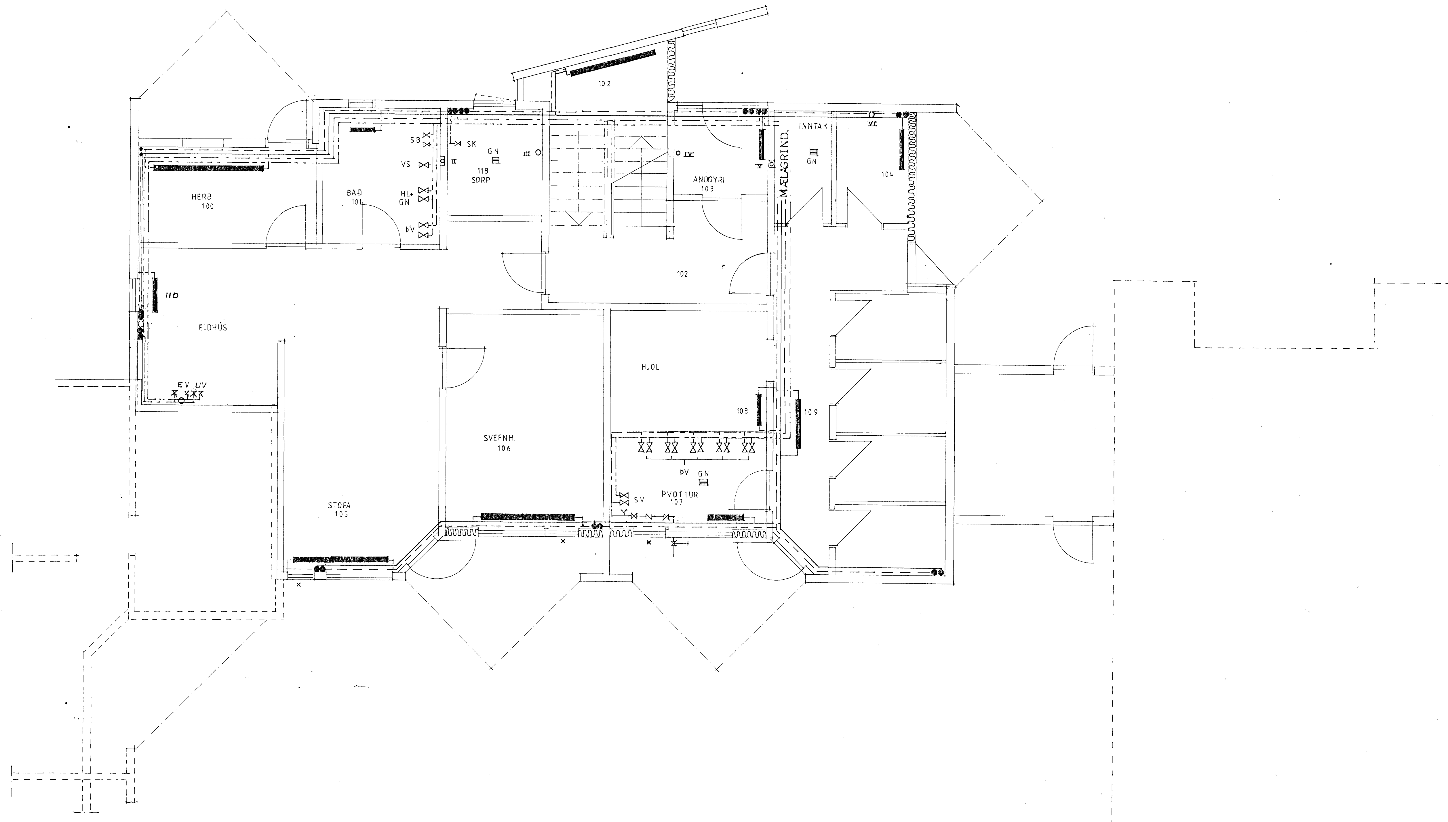
GRUNNMYND 1.HÆÐAR 1:50
