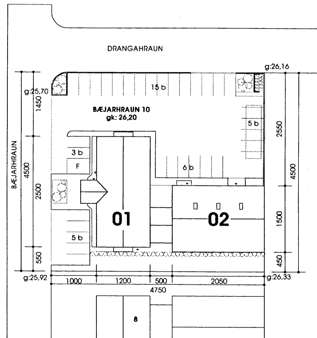
1 AFSTÖÐUMYND m.kv. 1:500
