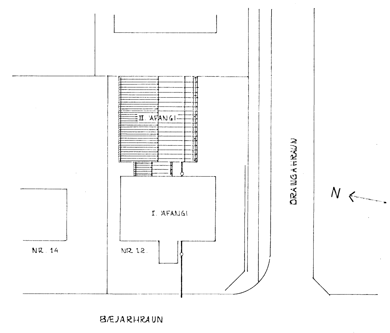
AFSTÖÐUMYND 1:500
