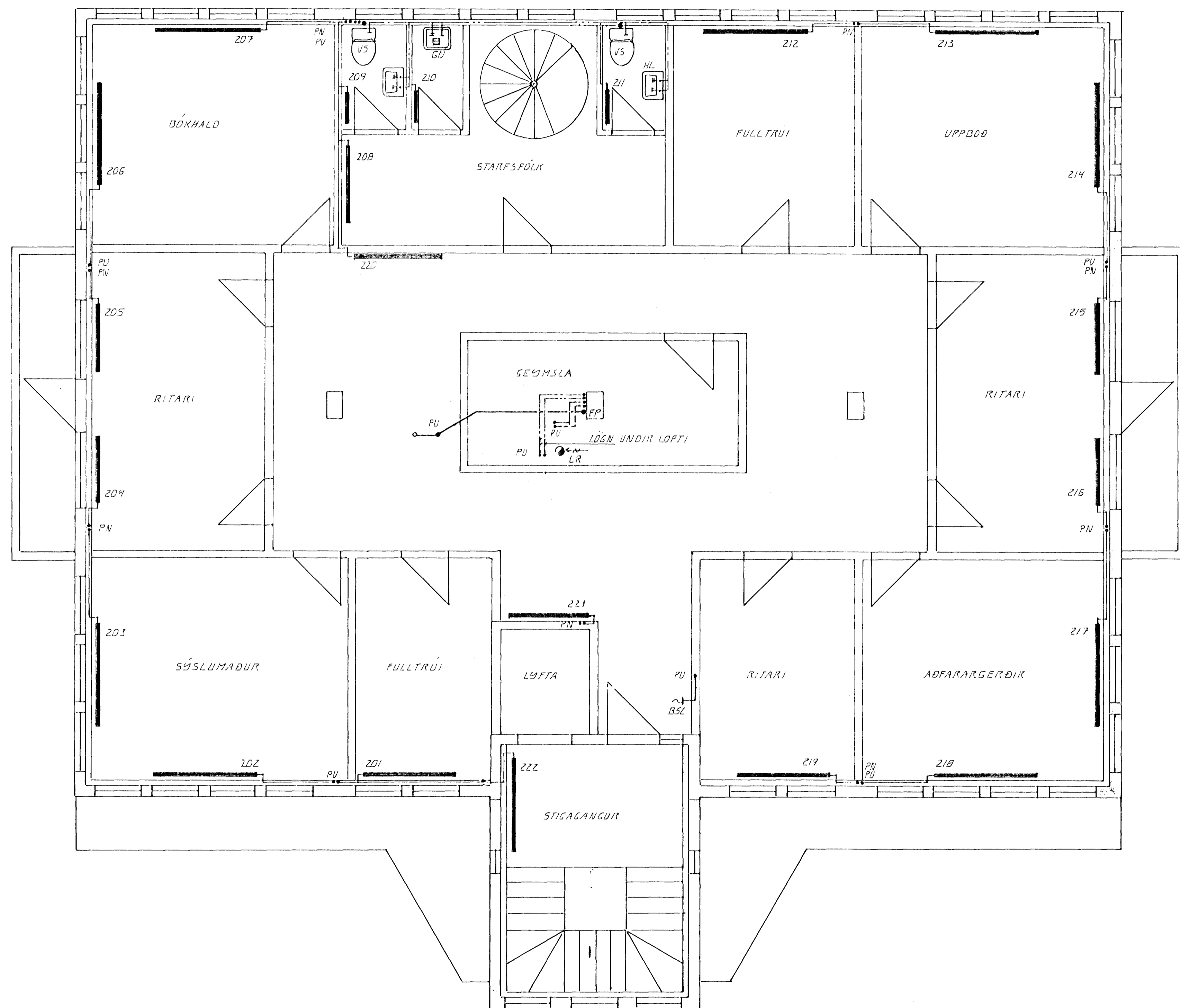
2. HÆÐ GRUNNMÝND. 1:50
