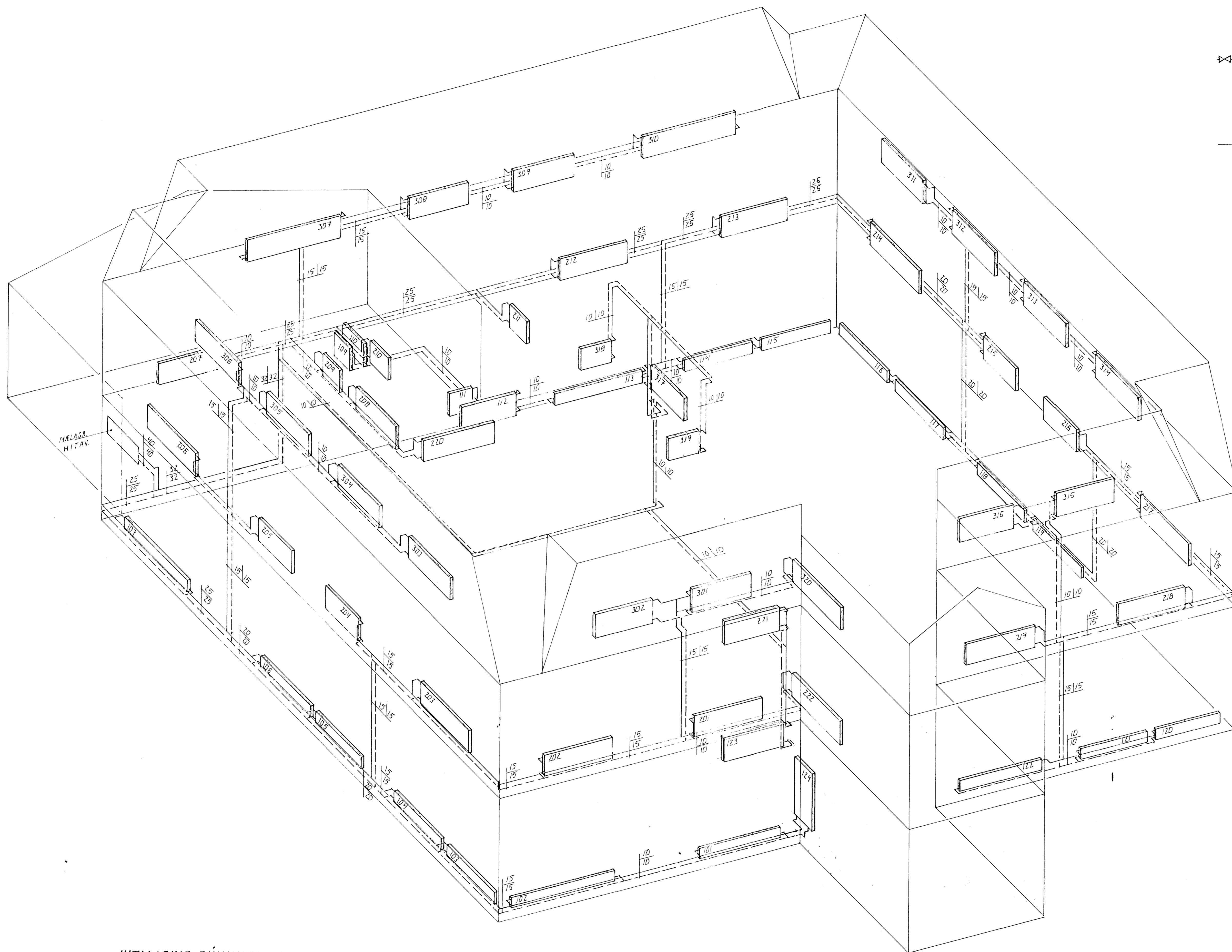
HITALAGNIK RÚMMYND, 1:50
