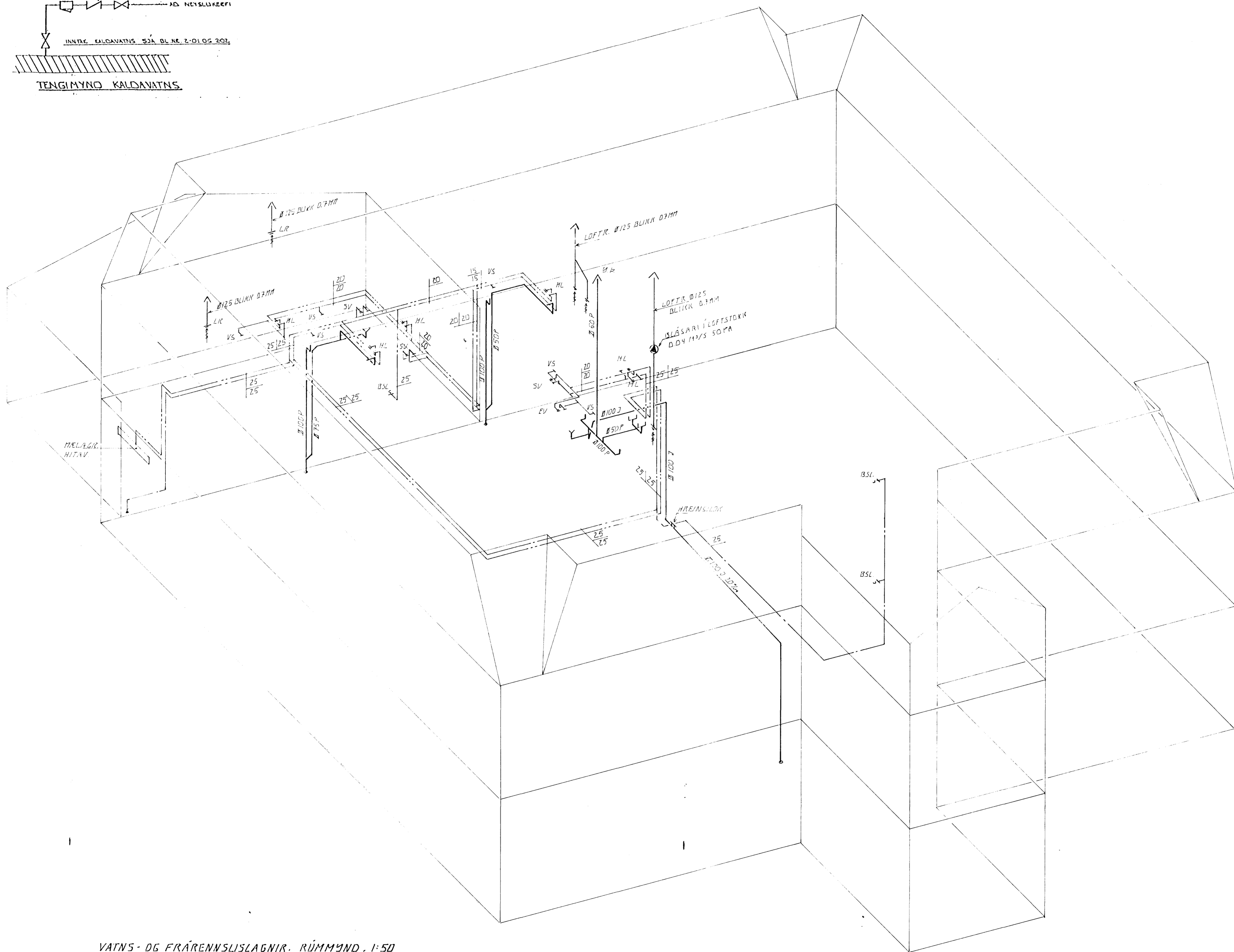
VATNS- OG FRÁRENNISLAGNIR. RÚMMYND. 1:50
