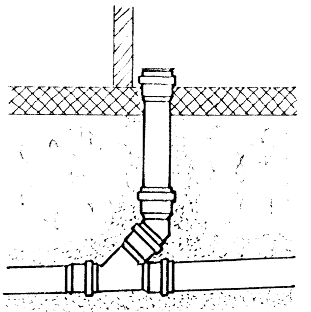
SÉRMYND A. HREINISSTÚTUR 150 PVC UPP Í GOLF
