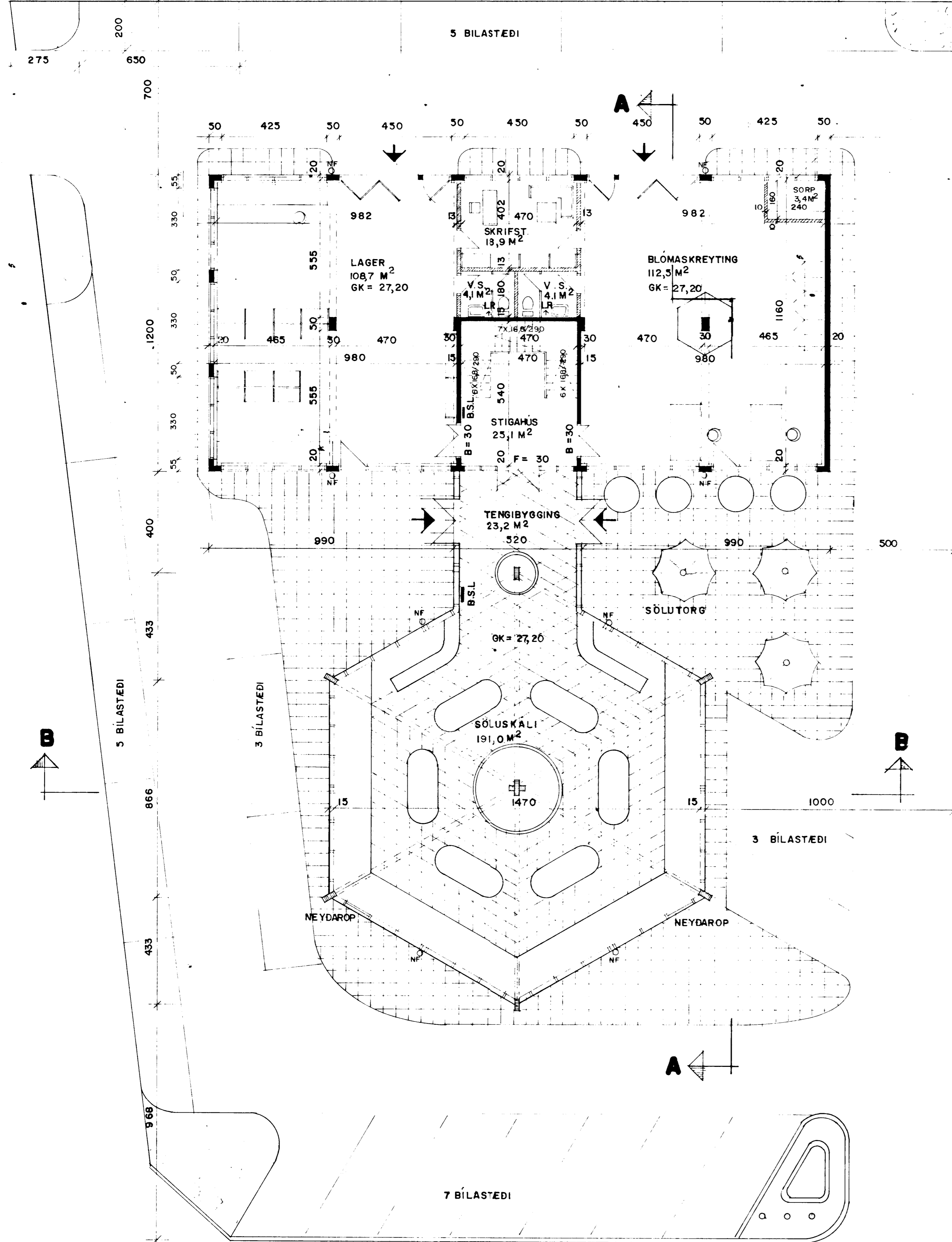
GRUNNMYND, I. HÆÐAR M. 1:100.
