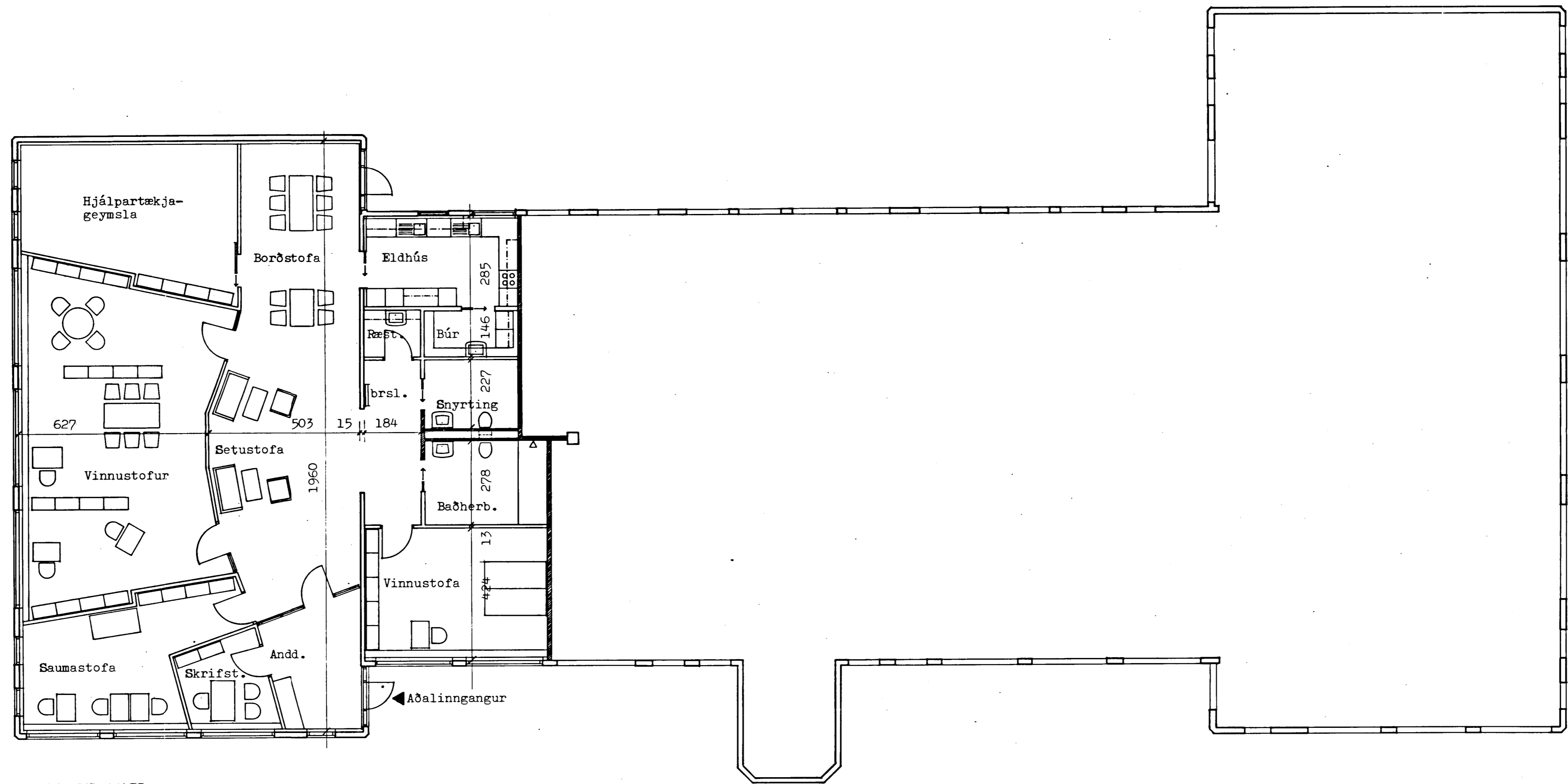
GRUNNMYND 1.HÆÐ
