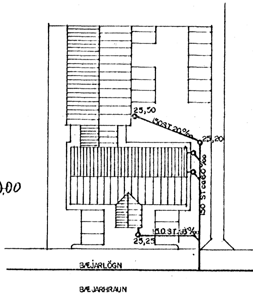
AFSTÖÐUMYND M. 1:500
