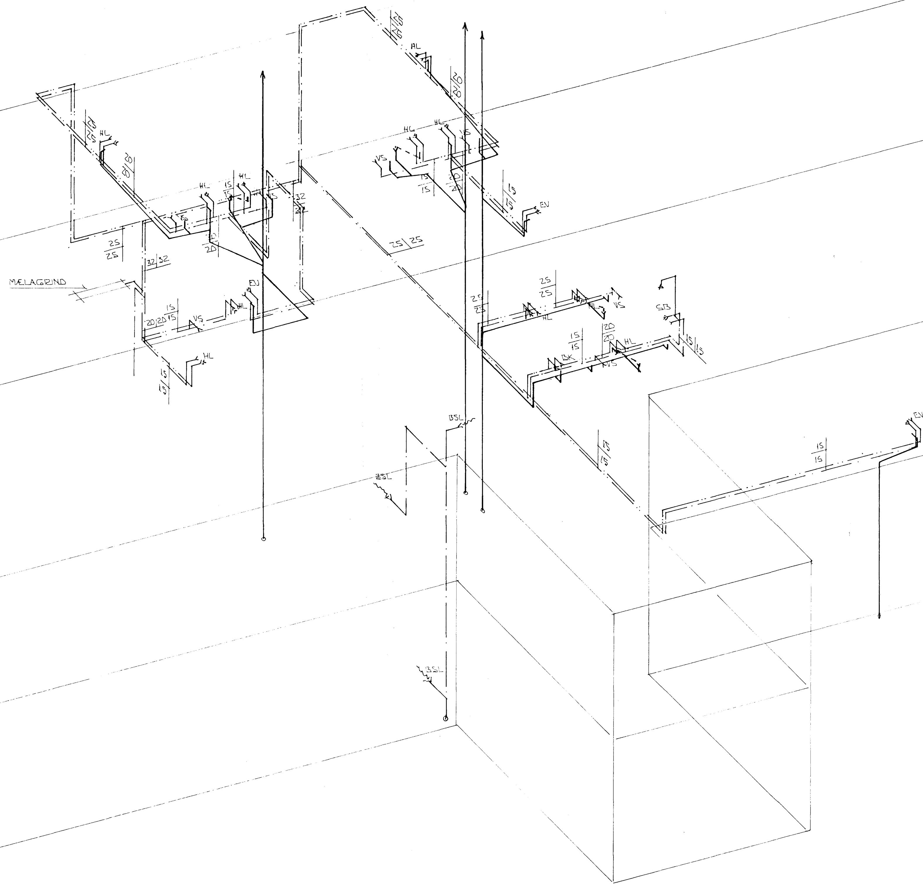
RÚMMYND VATNSLAGNA 1:50
