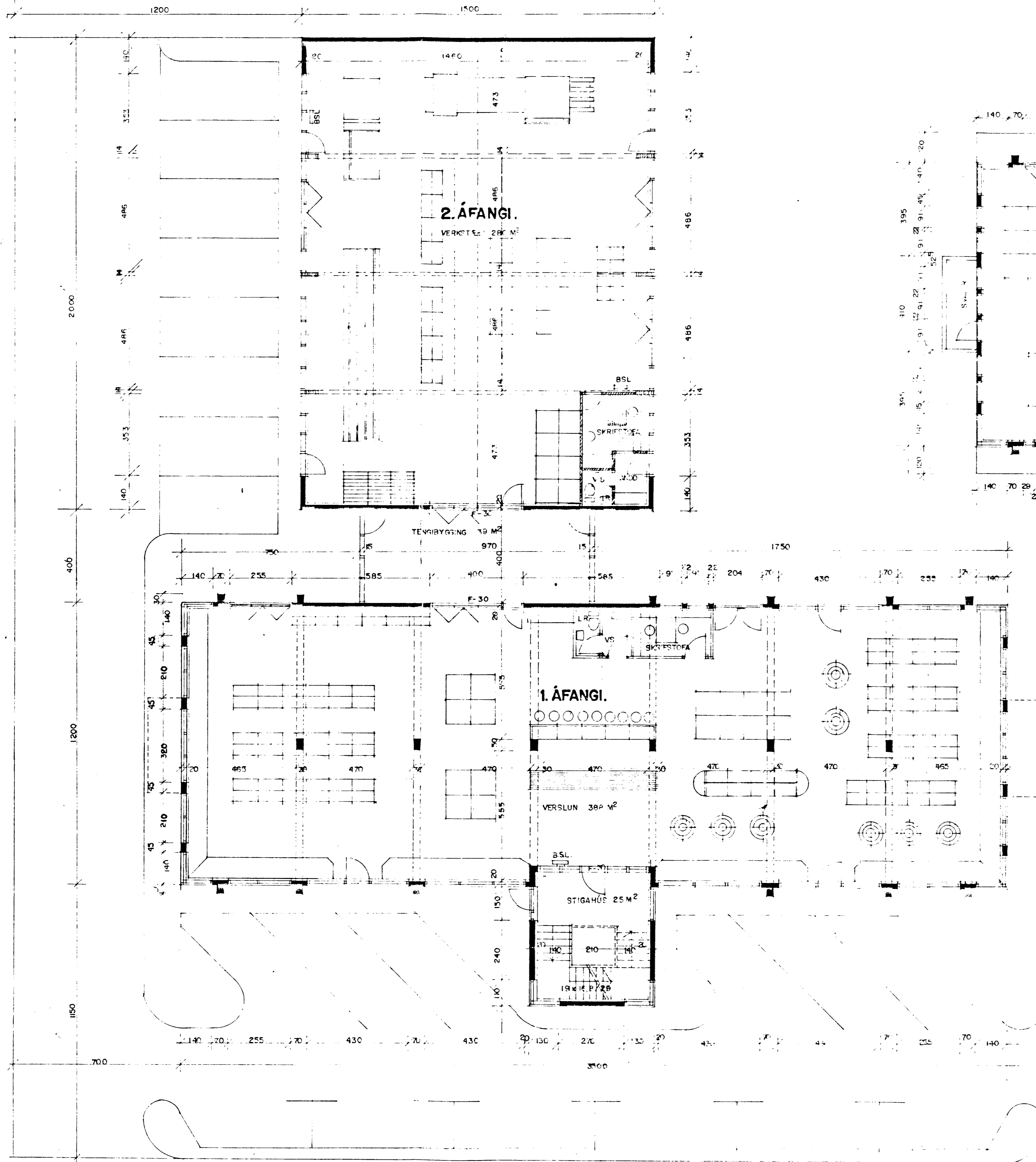
GRUNNMYND I. HÆÐ. M. 1:100.
