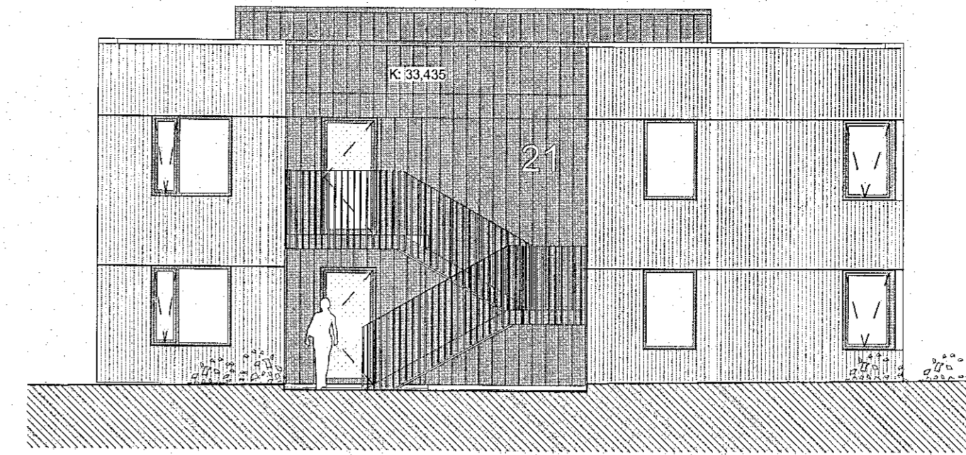
07-Norður punkthús - Mhl. 03 1:100
