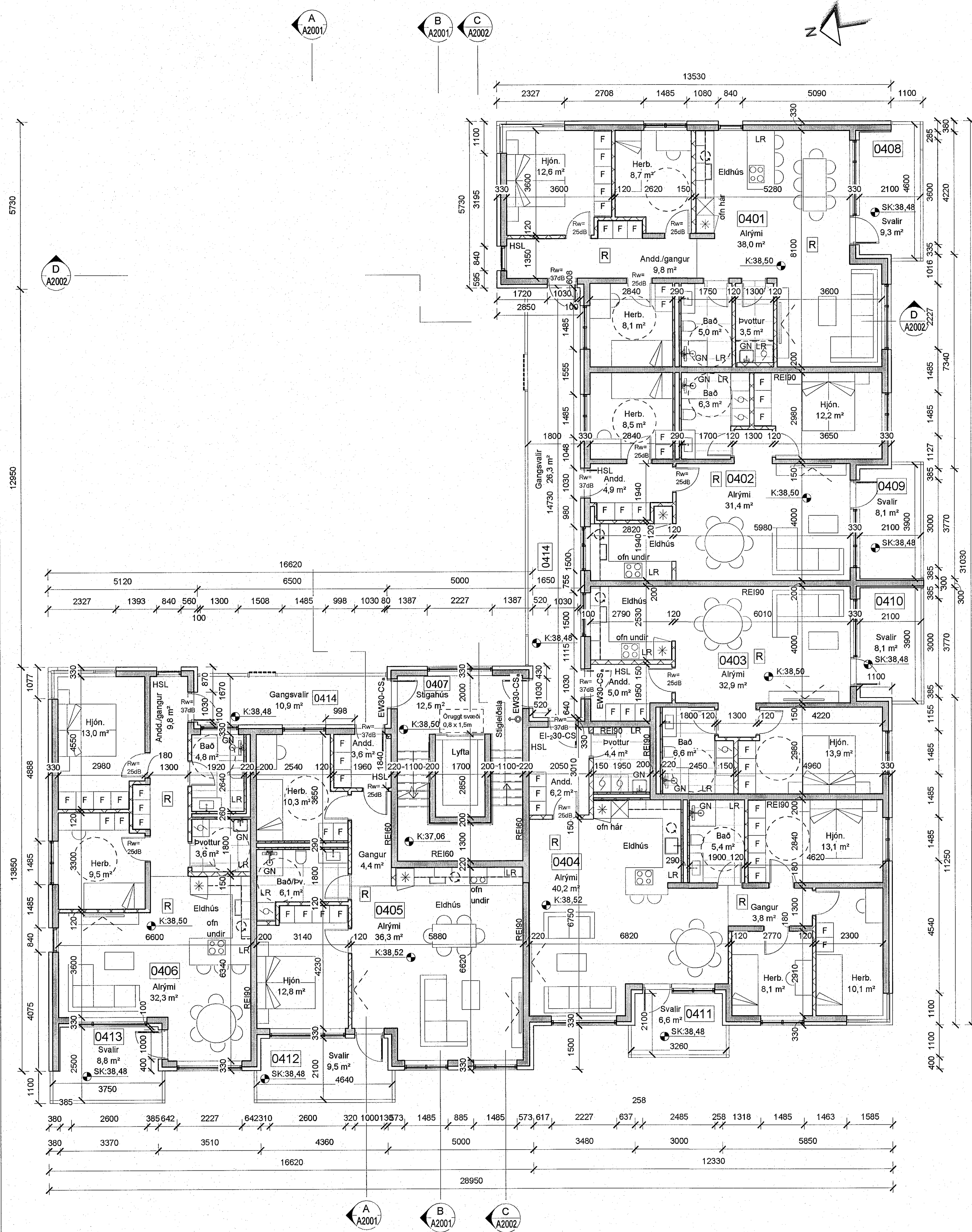
4.hæð mkv: 1 : 100
