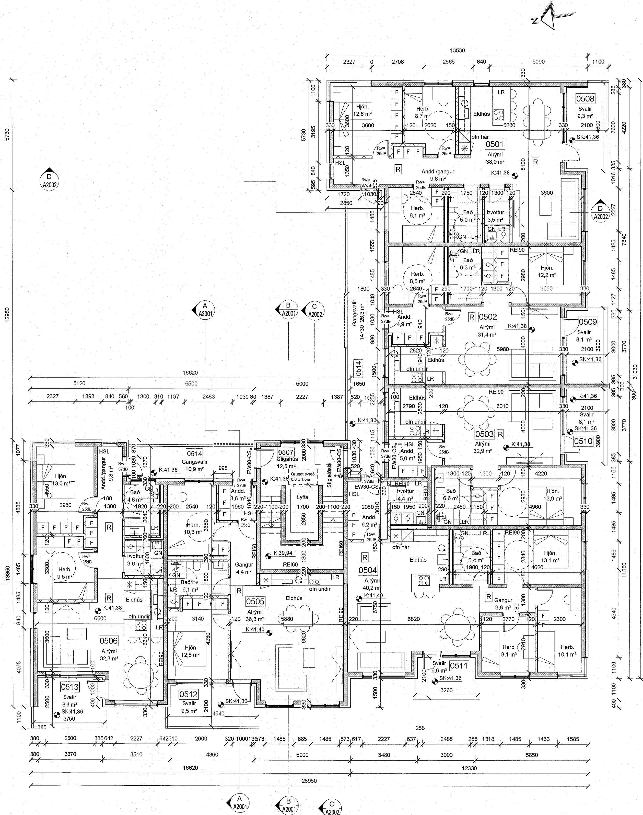
5.hæð mkv: 1 : 100
