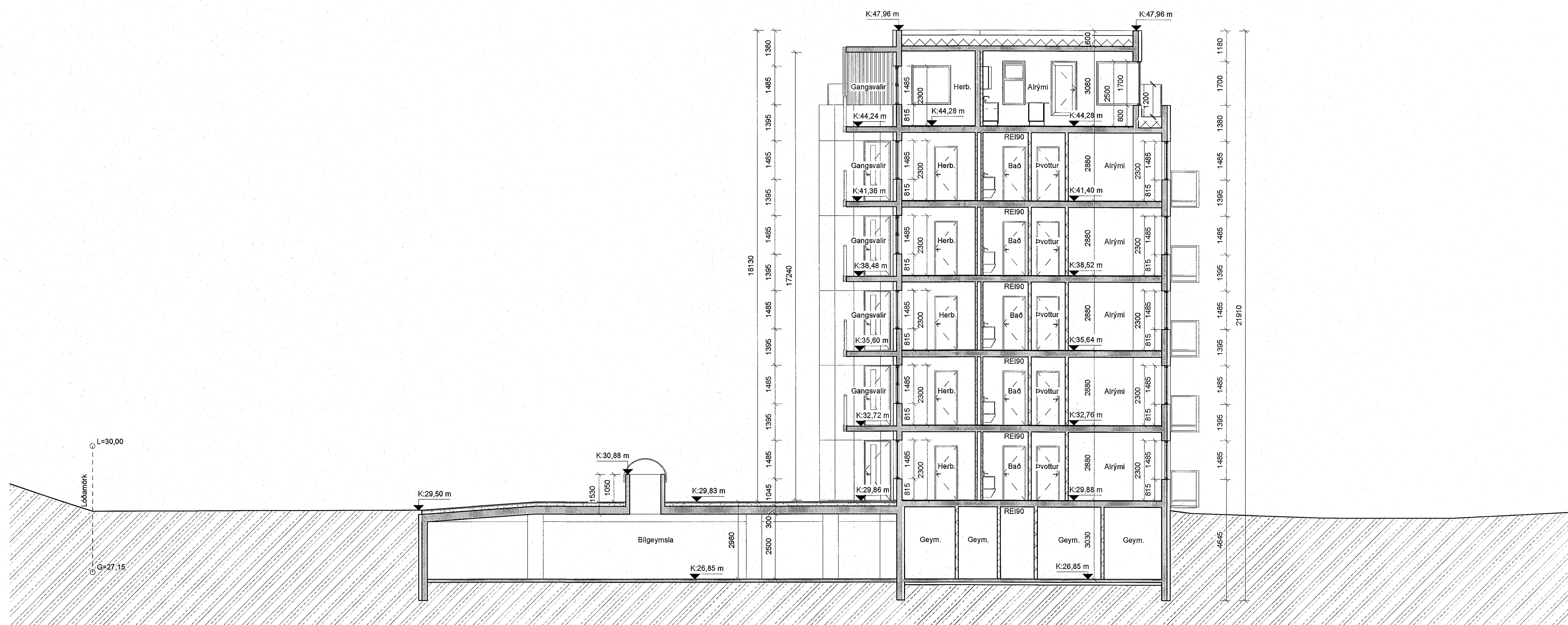
Snið D-D mkv: 1 : 100
