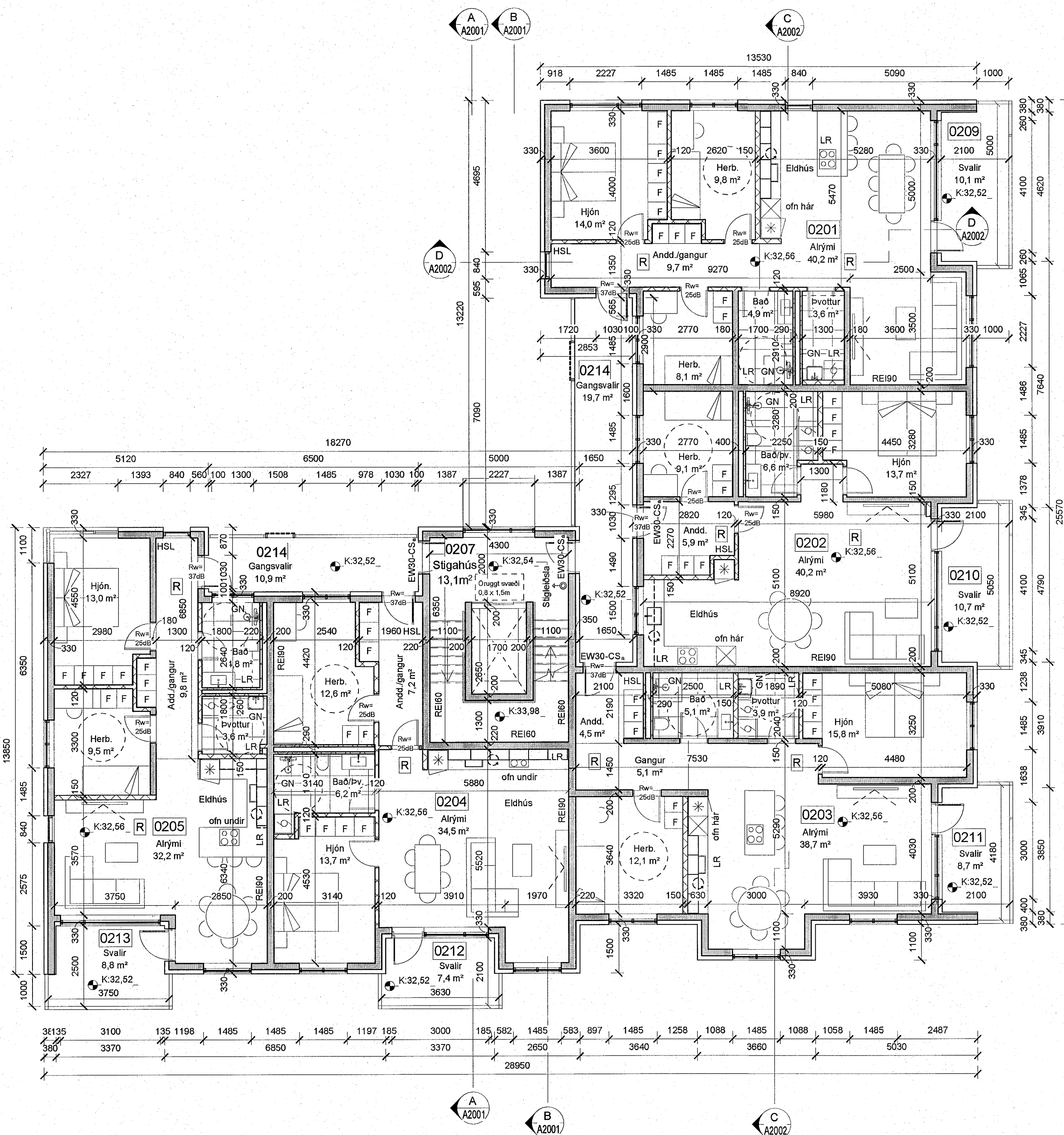
2.hæð mkv: 1 : 100
