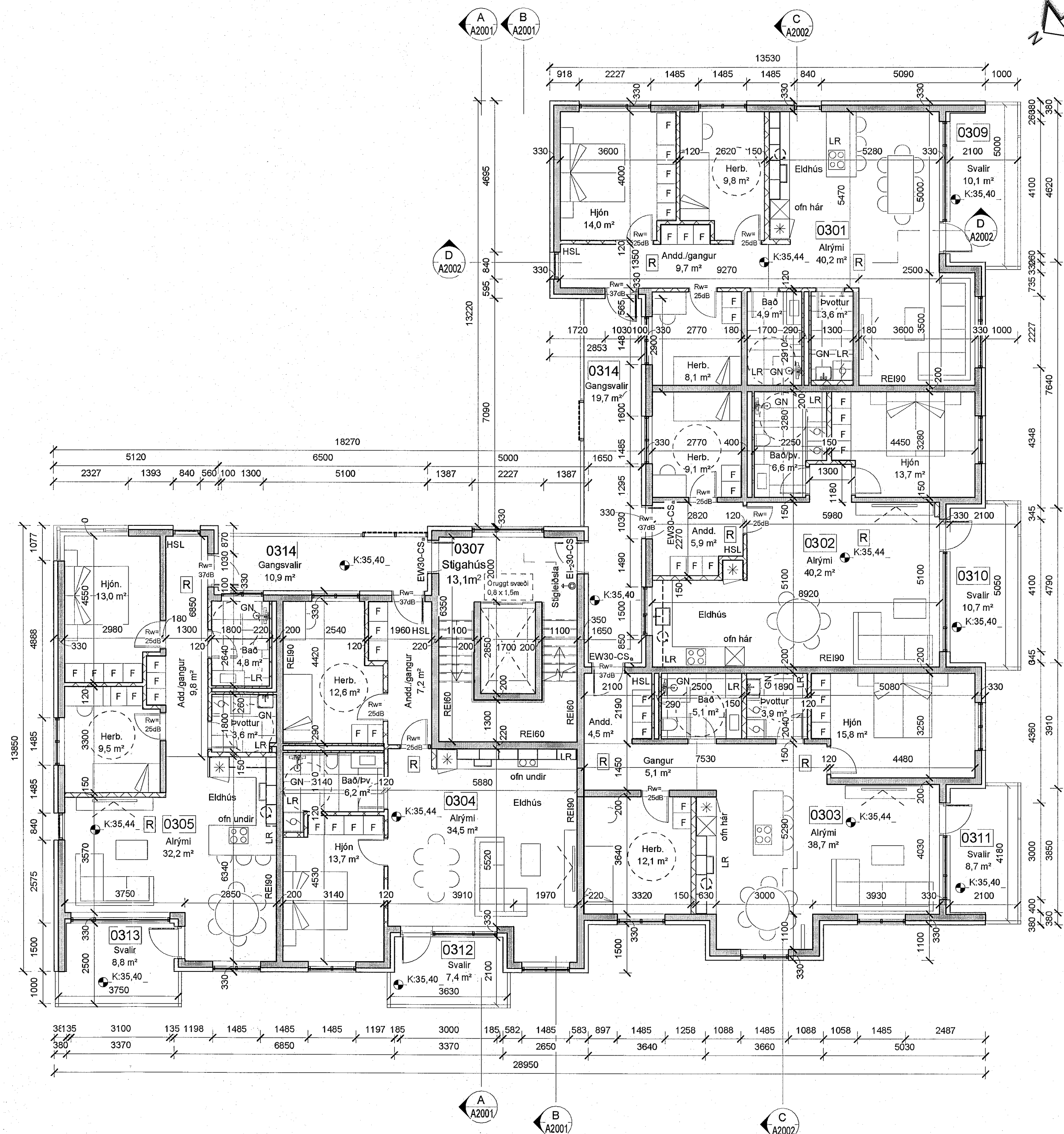
3.hæð mkv: 1 : 100
