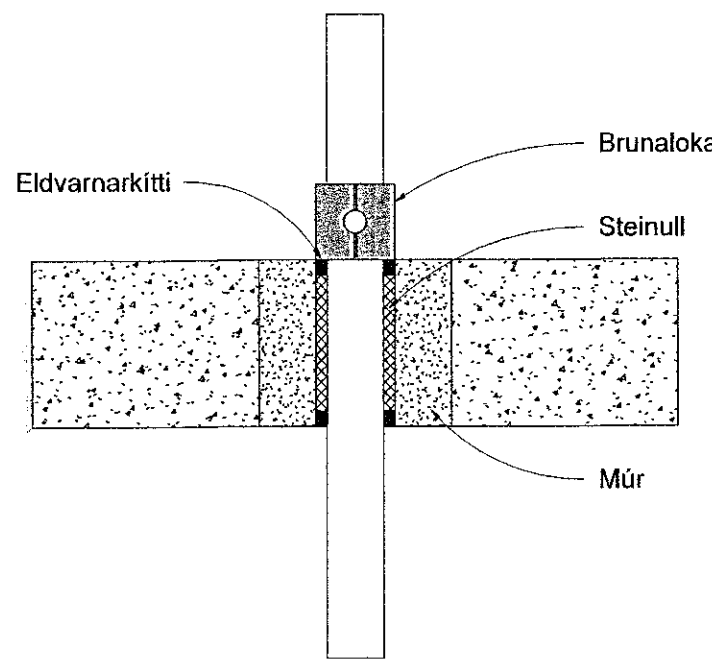
Brunapétting á loftræstilögn í gegnum steipt gólf utan lagnaskakts
