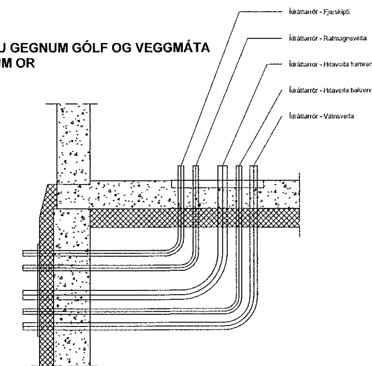
FRÁGANGUR INNTÖK VEITNA [1:20]
