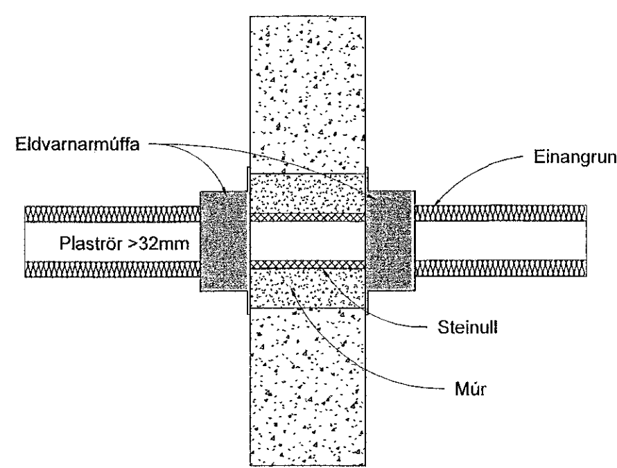
Brunapétting á plastlögn stærri en Ø32mm í gegnum steiptan vegg
