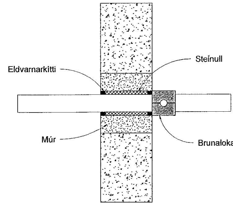
Brunapétting á loftræstilögn í gegnum steiptan vegg
