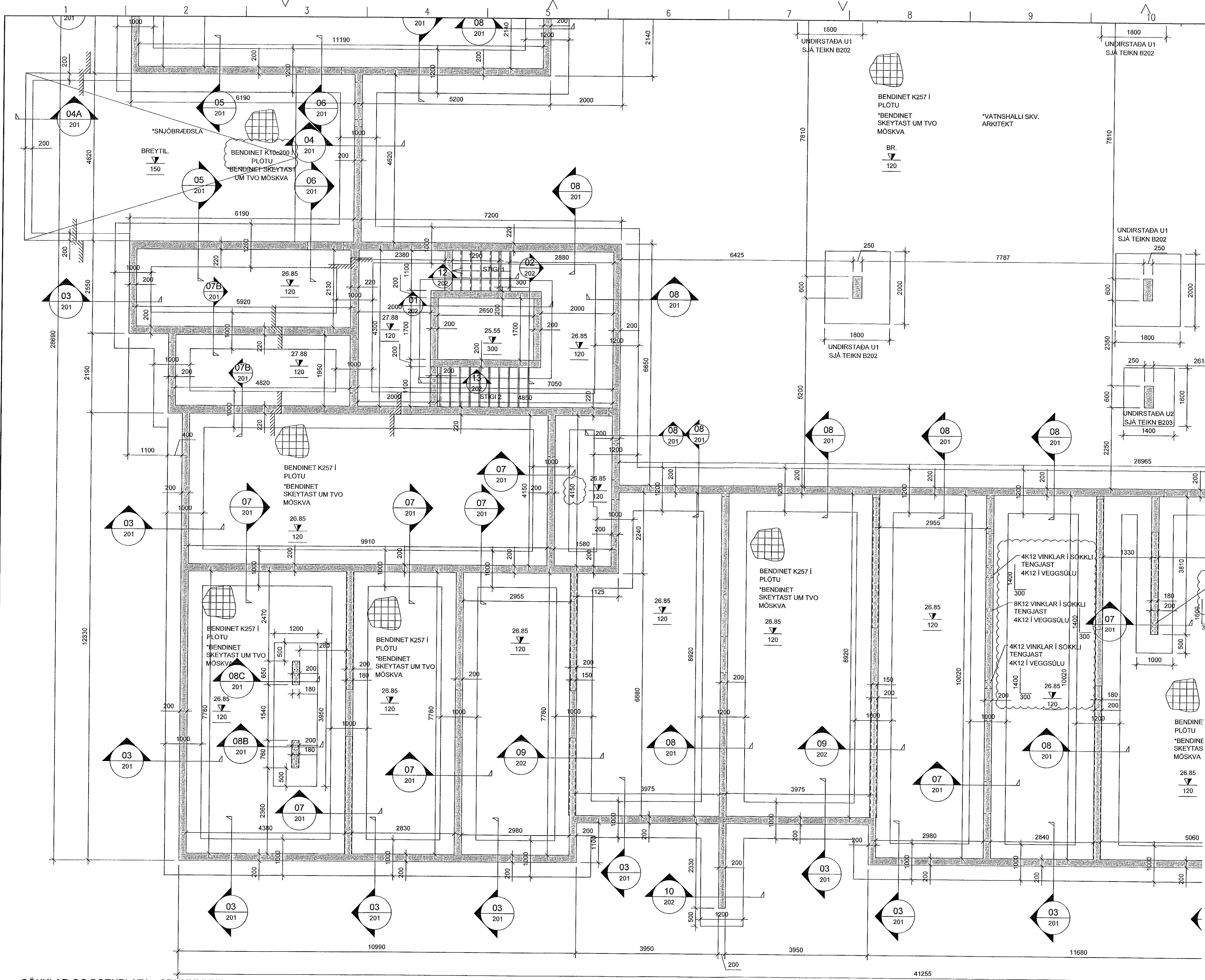
SÖKKLAR OG BOTNPLATA, GRUNNMÝND MKV. 3
