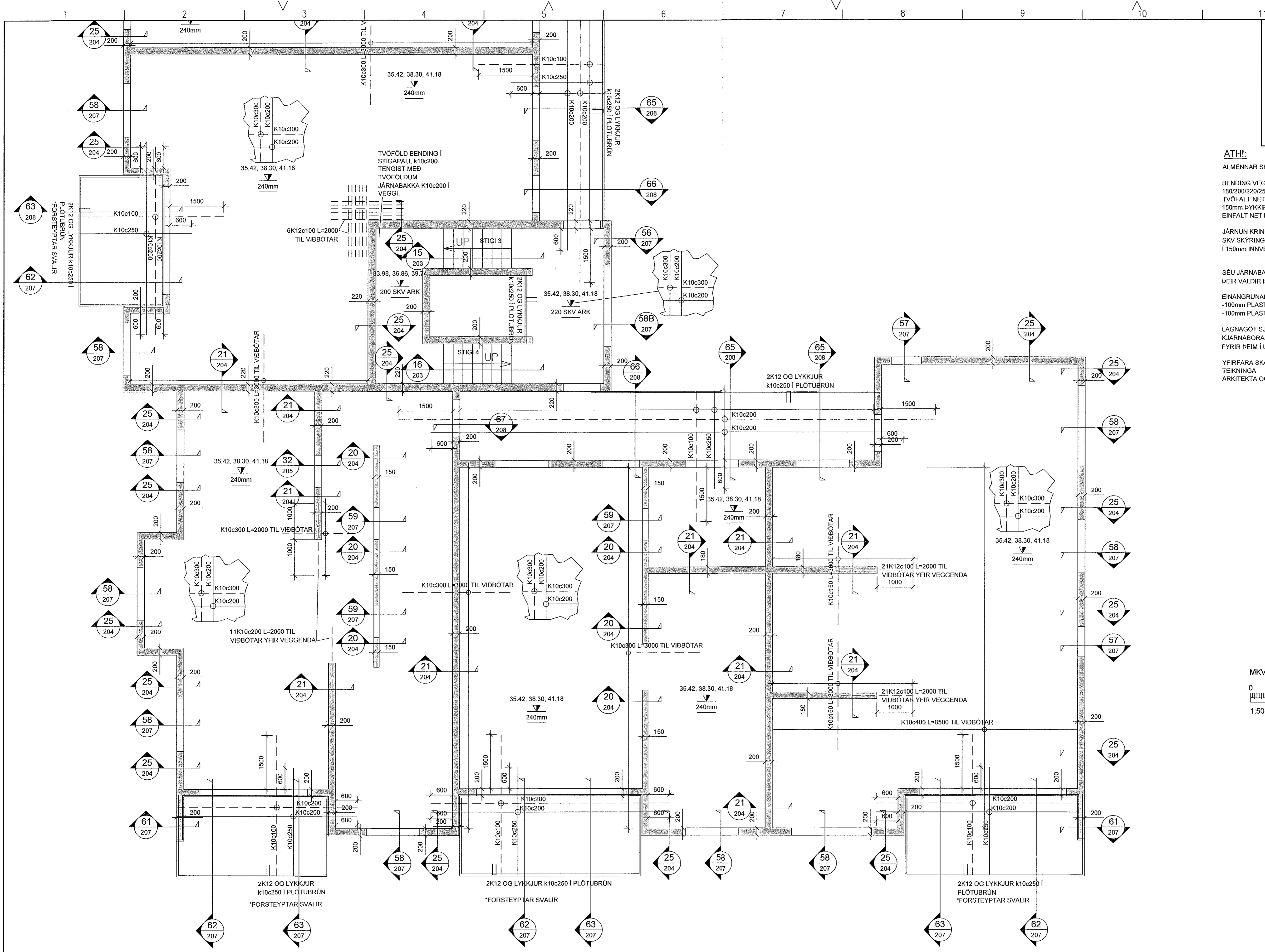
VEGGIR OG LOFTAPLATA 2, 3, 4 HÆÐAR, GRUNNMÝND MKV. 3
