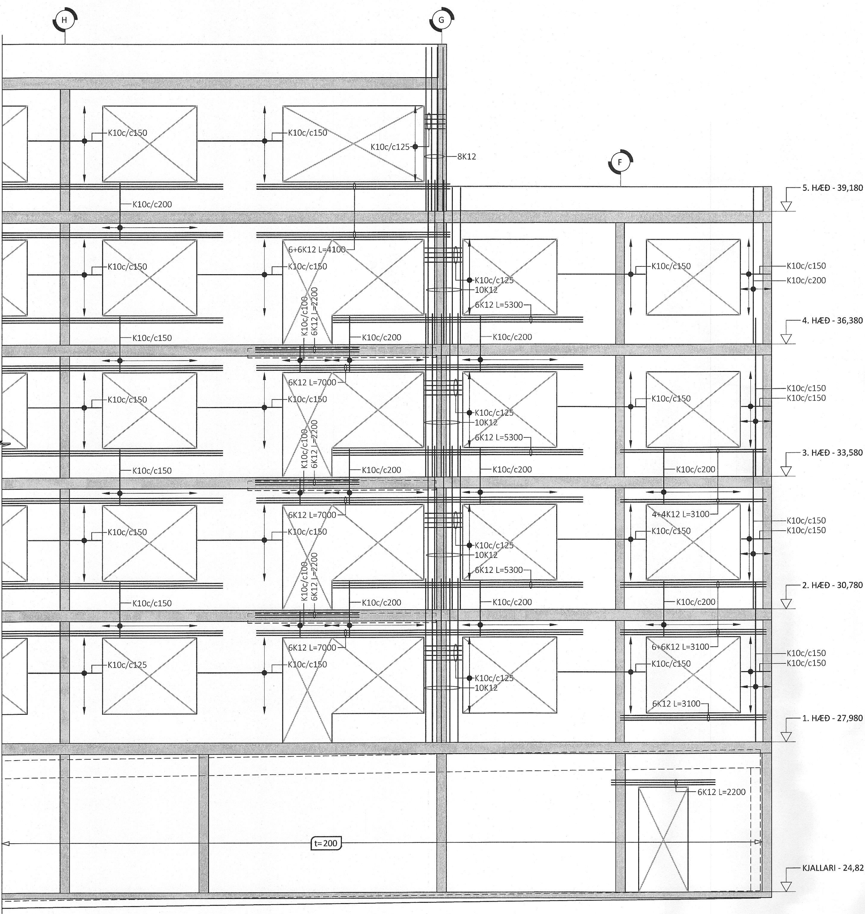
HLIÐARMYND VEGGIJAR V009 - M1:50: ÞYKKT VEGGIJAR: 180mm NEMA ANNAD SÉ SÉRSTAKLEGA TEKID FRAM
