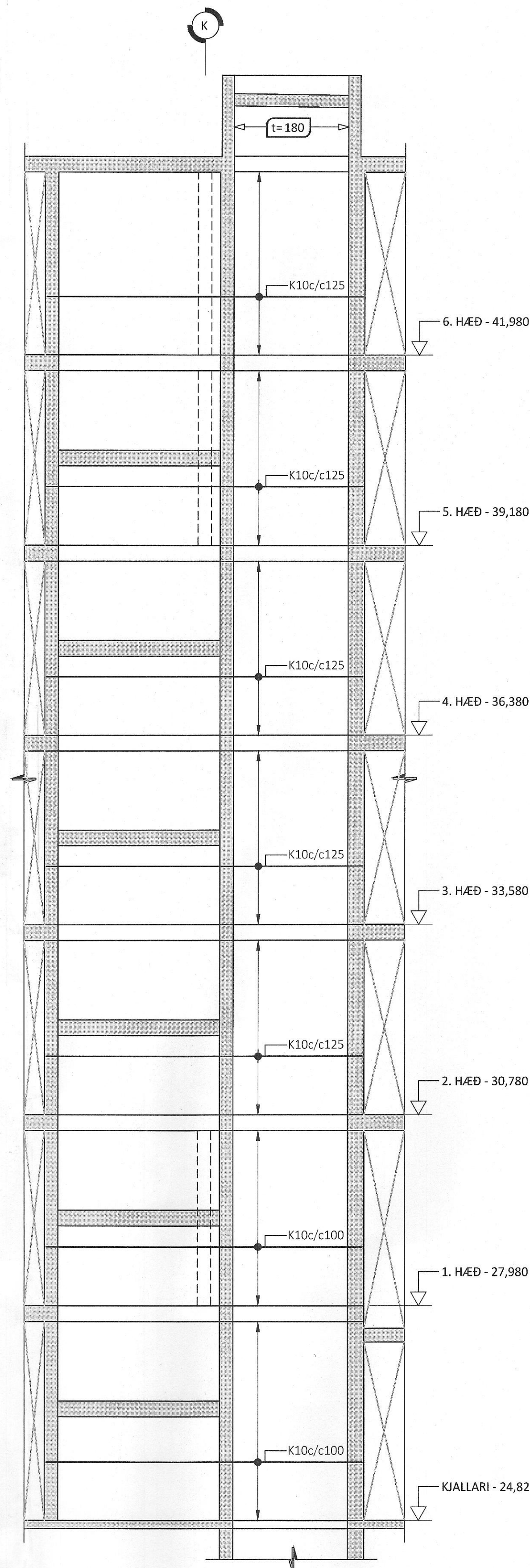
HLIÐARMYND VEGGIJAR V010 - M1:50: ÞYKKT VEGGIJAR: 240mm NEMA ANNAD SÉ SÉRSTAKLEGA TEKID FRAM
