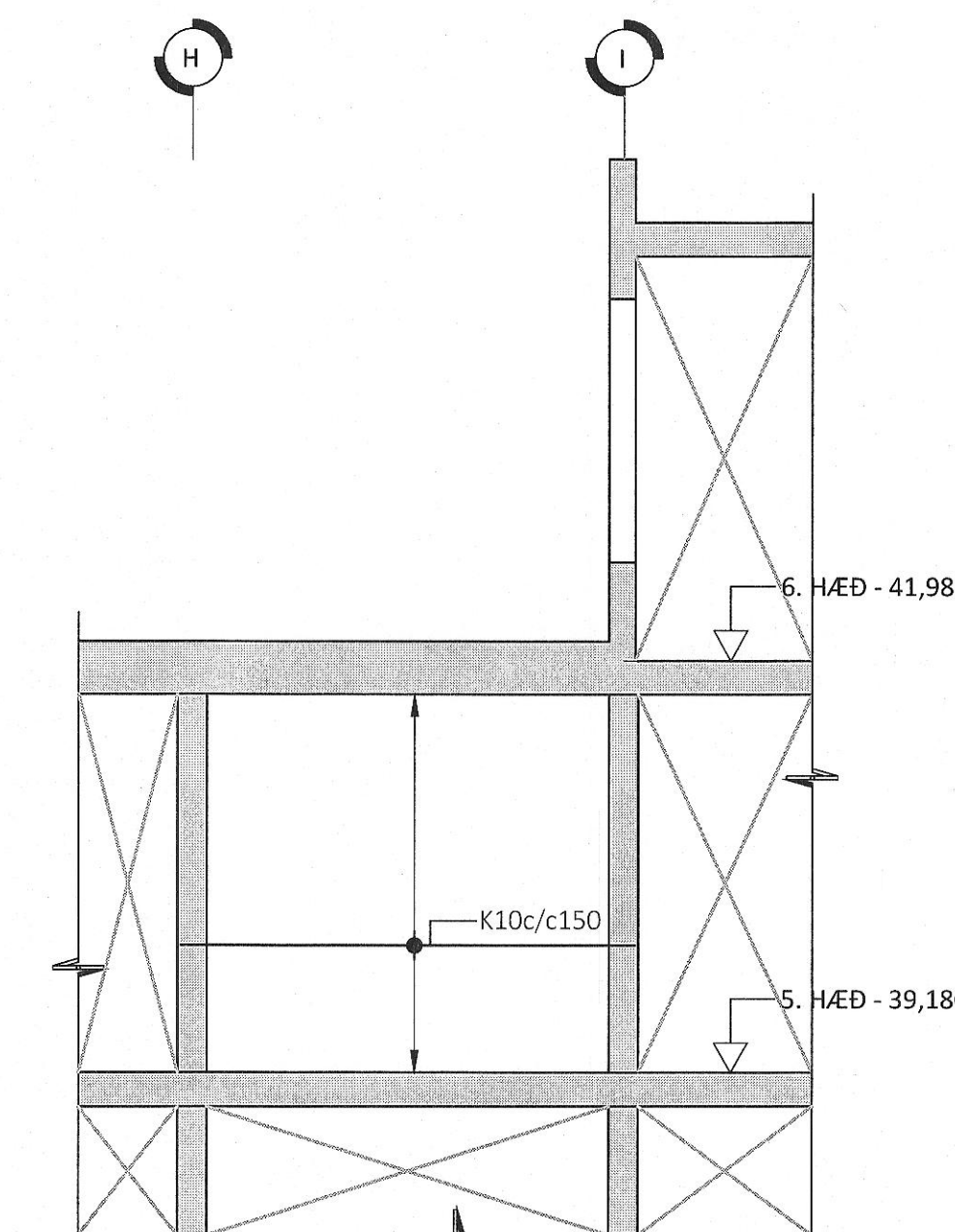
HLIÐARMYND VEGGIJAR V011 - M1:50: ÞYKKT VEGGIJAR: 200mm
