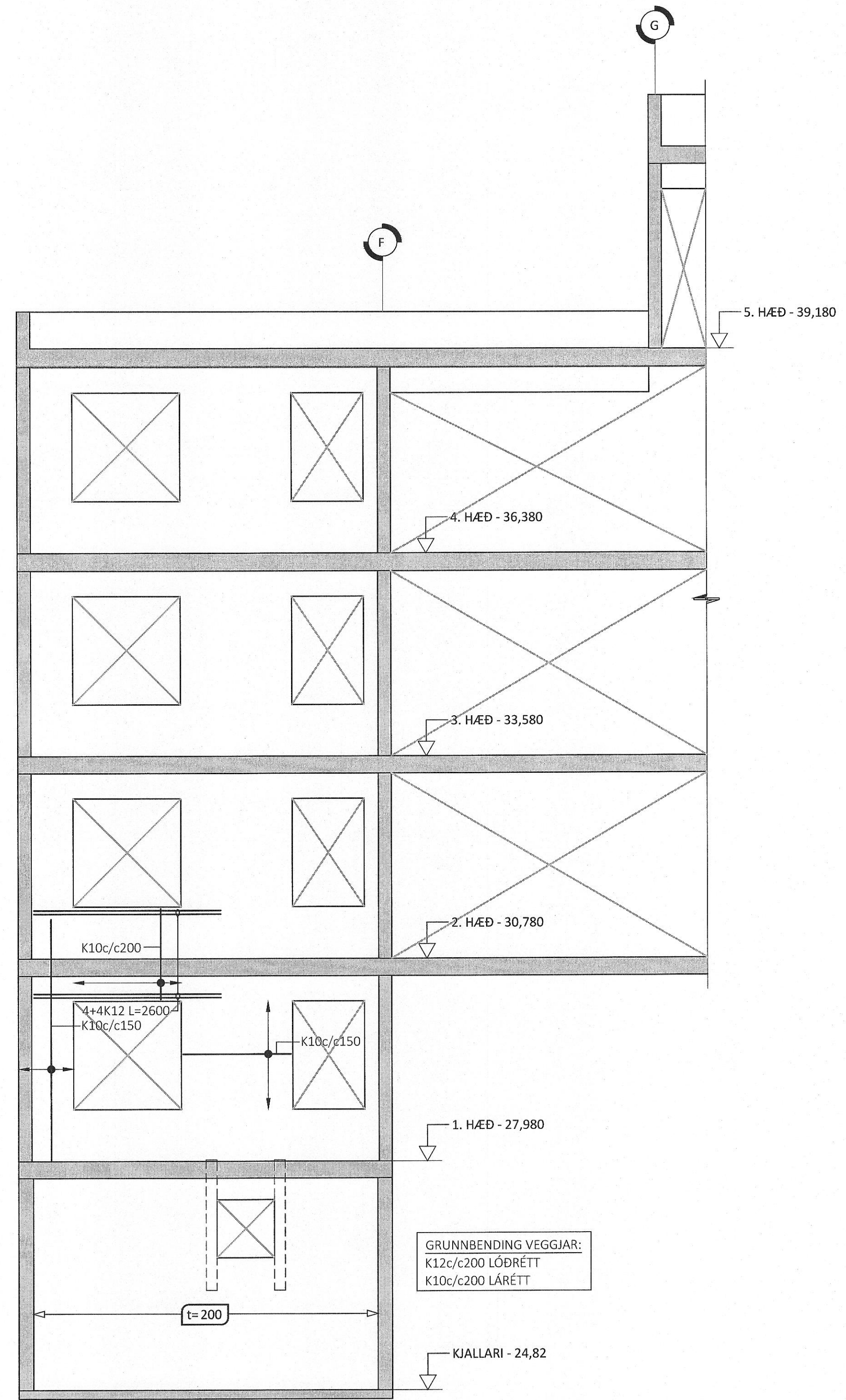
HLIÐARMYND VEGGIAR V014 - M1:50: ÞYKKT VEGGIAR: 180mm NEMA ANNAD SÉ SÉRSTAKLEGA TEKID FRAM
