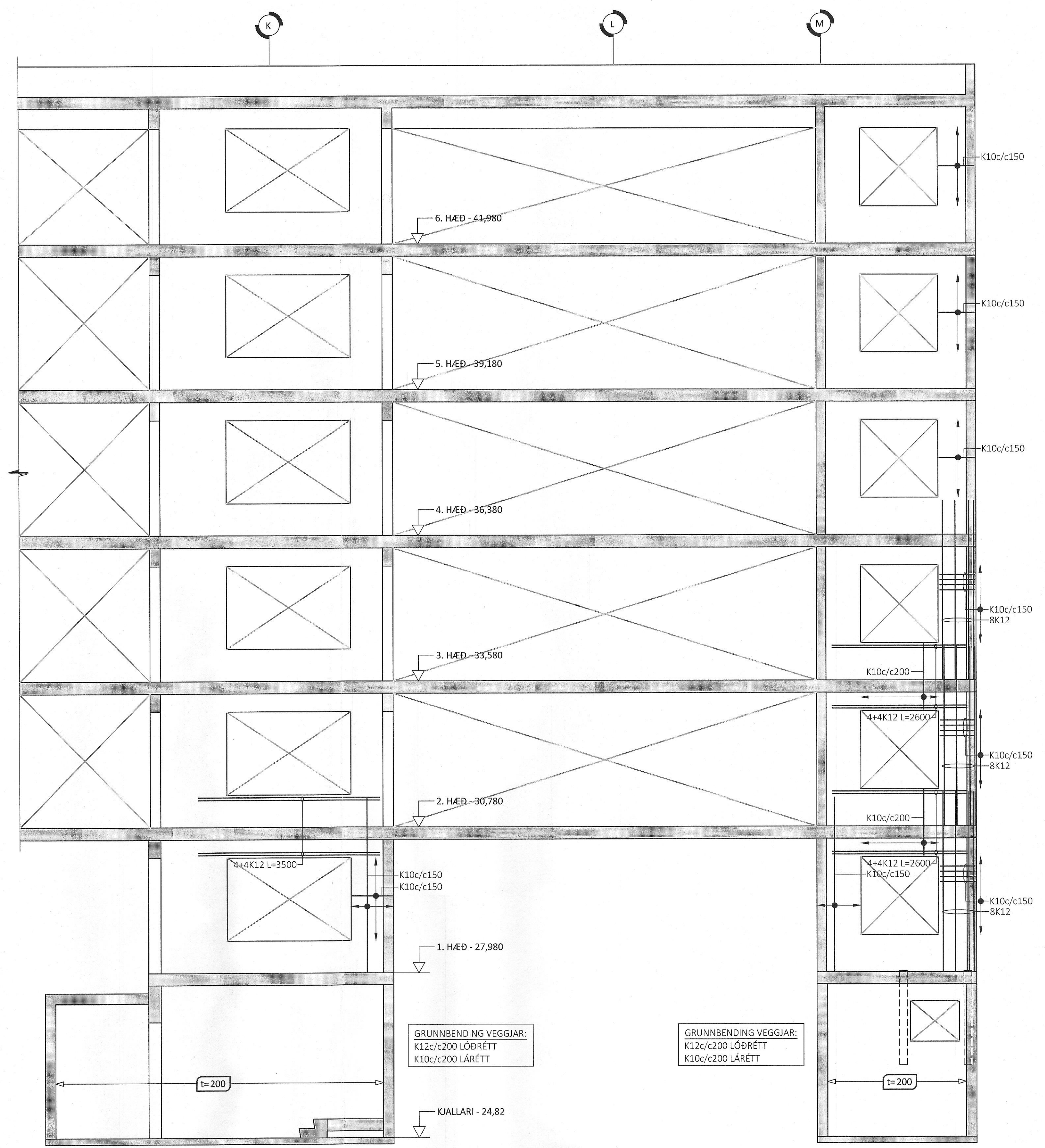
HLIÐARMYND VEGGIAR V015 - M1:50: ÞYKKT VEGGIAR: 180mm NEMA ANNAD SÉ SÉRSTAKLEGA TEKID FRAM
