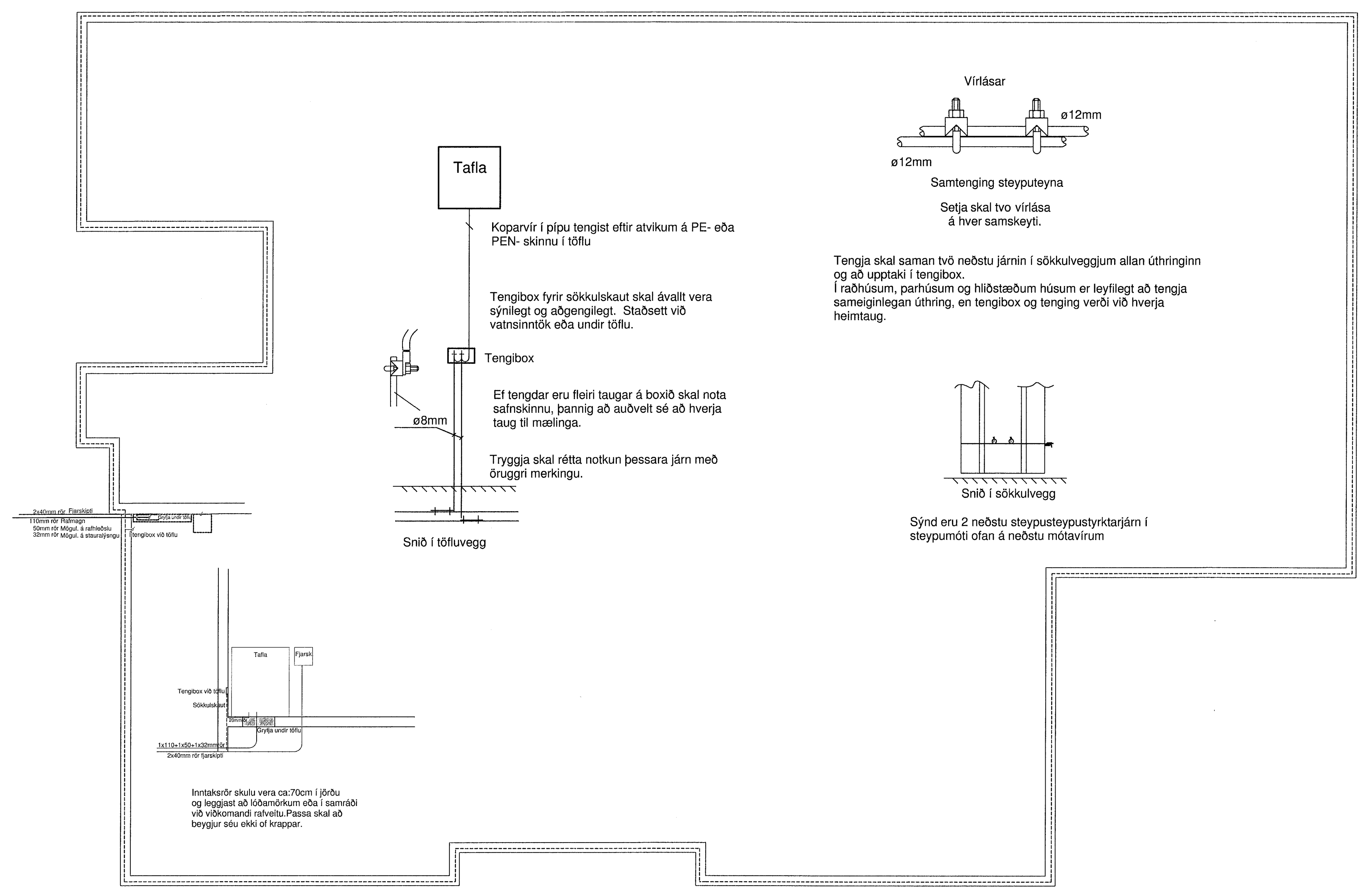
Sökkulskaut - Heimtaugar 1:100
