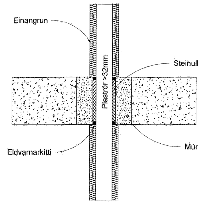
Brunapétting á plastlögn stærri en Ø32mm í gegnum steypnt gólf innan lagnaskakts
