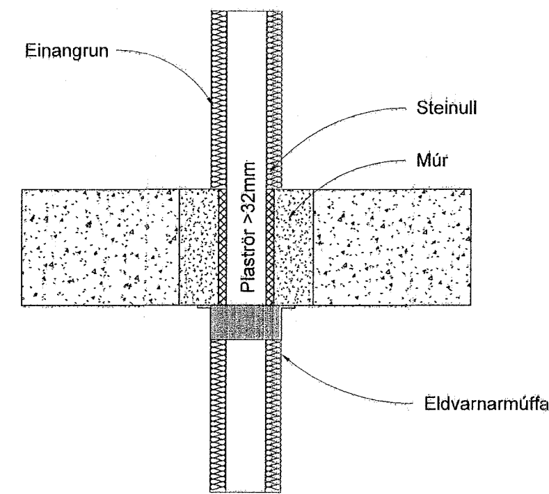
Brunapétting á plastlögn stærri en Ø32mm í gegnum steypnt gólf
