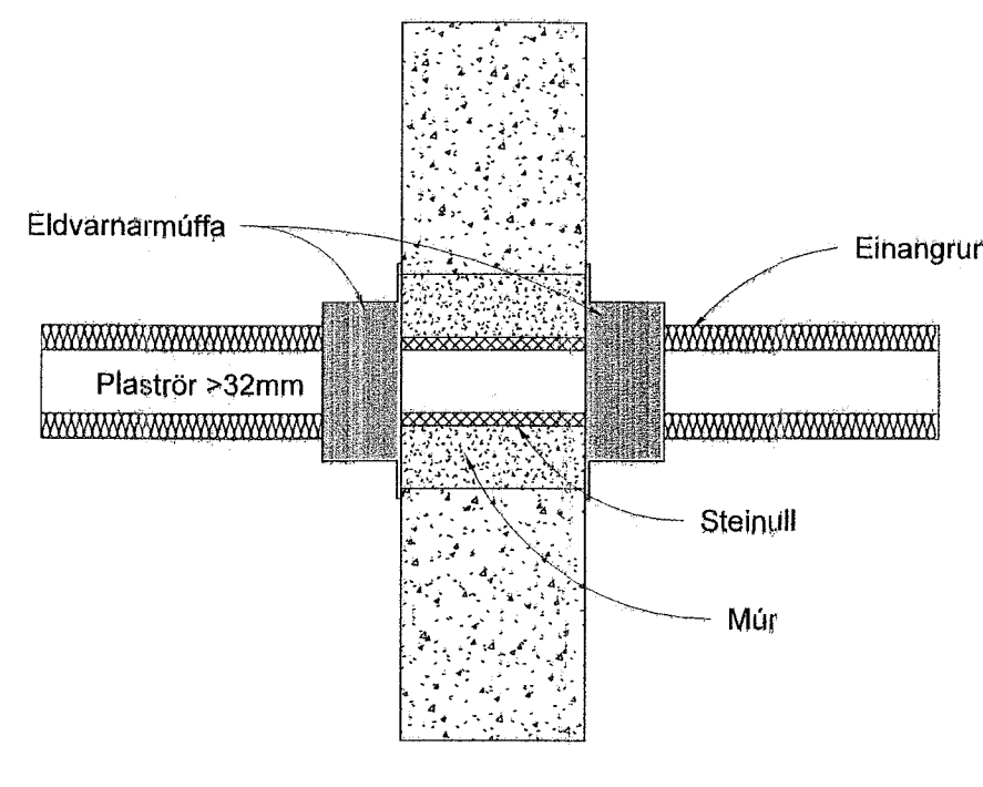
Brunapétting á plastlögn stærri en Ø32mm í gegnum steypnan vegg
