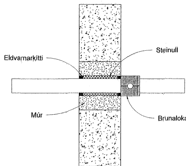
Brunapétting á loftræstilögn í gegnum steypnan vegg
