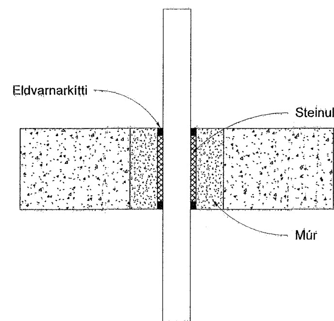
Brunapétting á loftræstilögn í gegnum steypnt gólf í lagnaskakti
