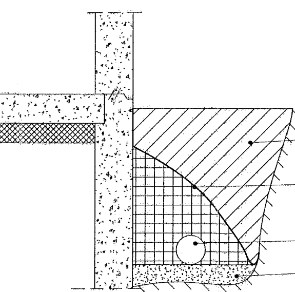
FRÁGANGUR DRENLAGNAR [1:20]
