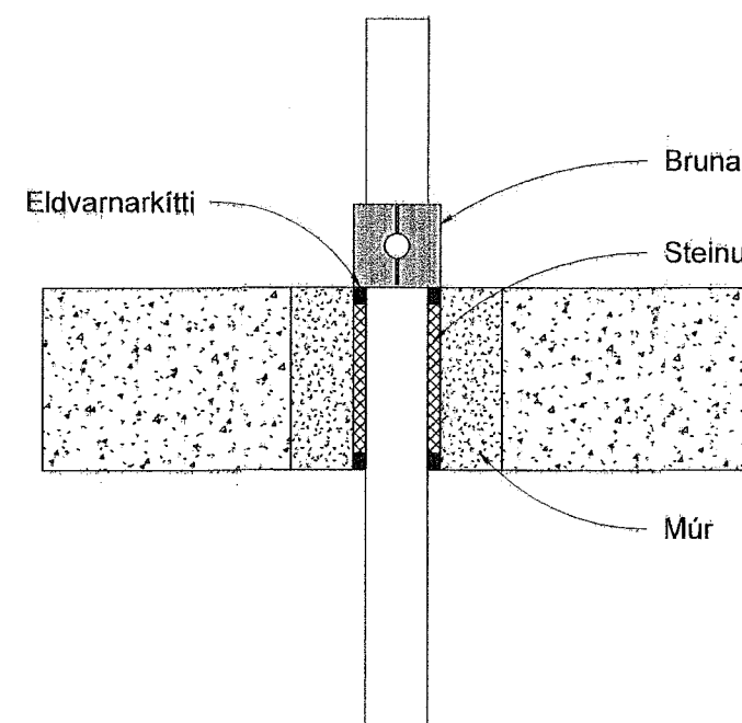
Brunapétting á loftræstilögn í gegnum steypnt gólf utan lagnaskakts
