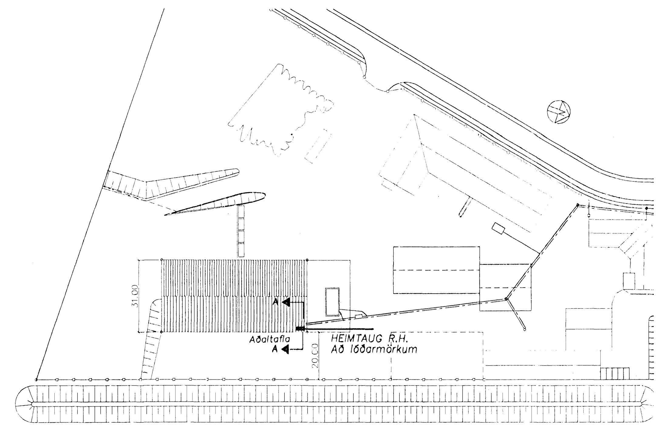
AFSTÖÐUMYND-INNTAK M.1:1000
