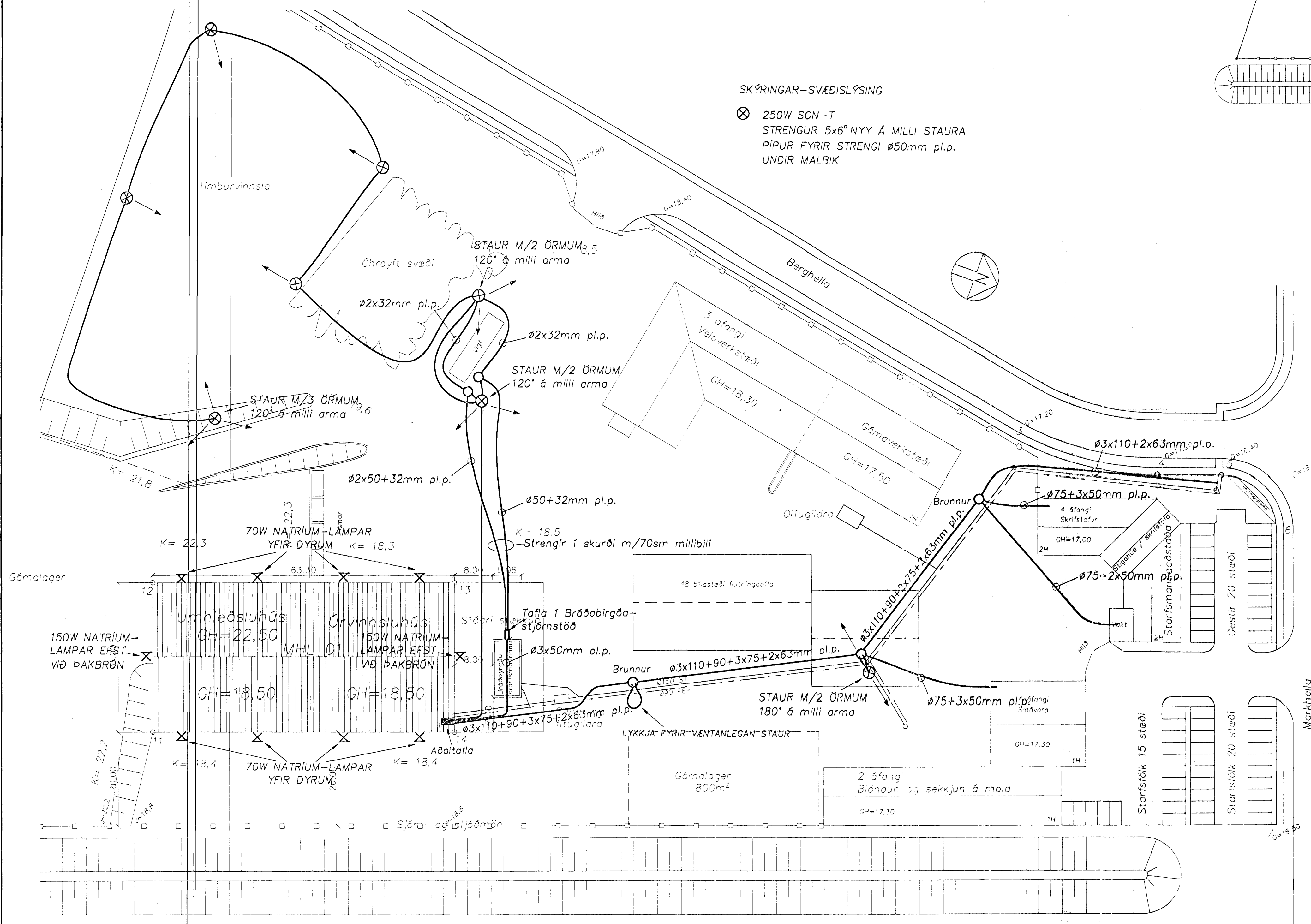
PIPUR Í JÖRÐU/SVÆÐISLÝSING M.1:500
