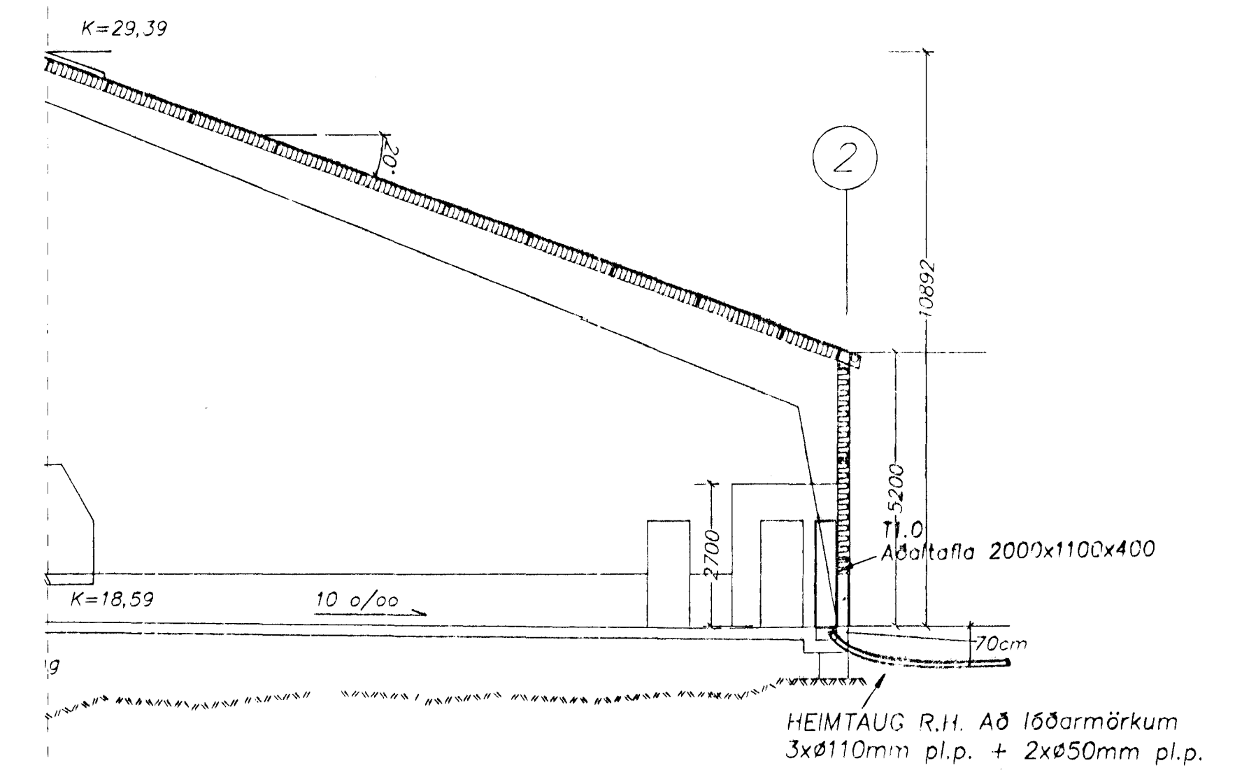
SNÍÐ Í INNTAK M.1:100
