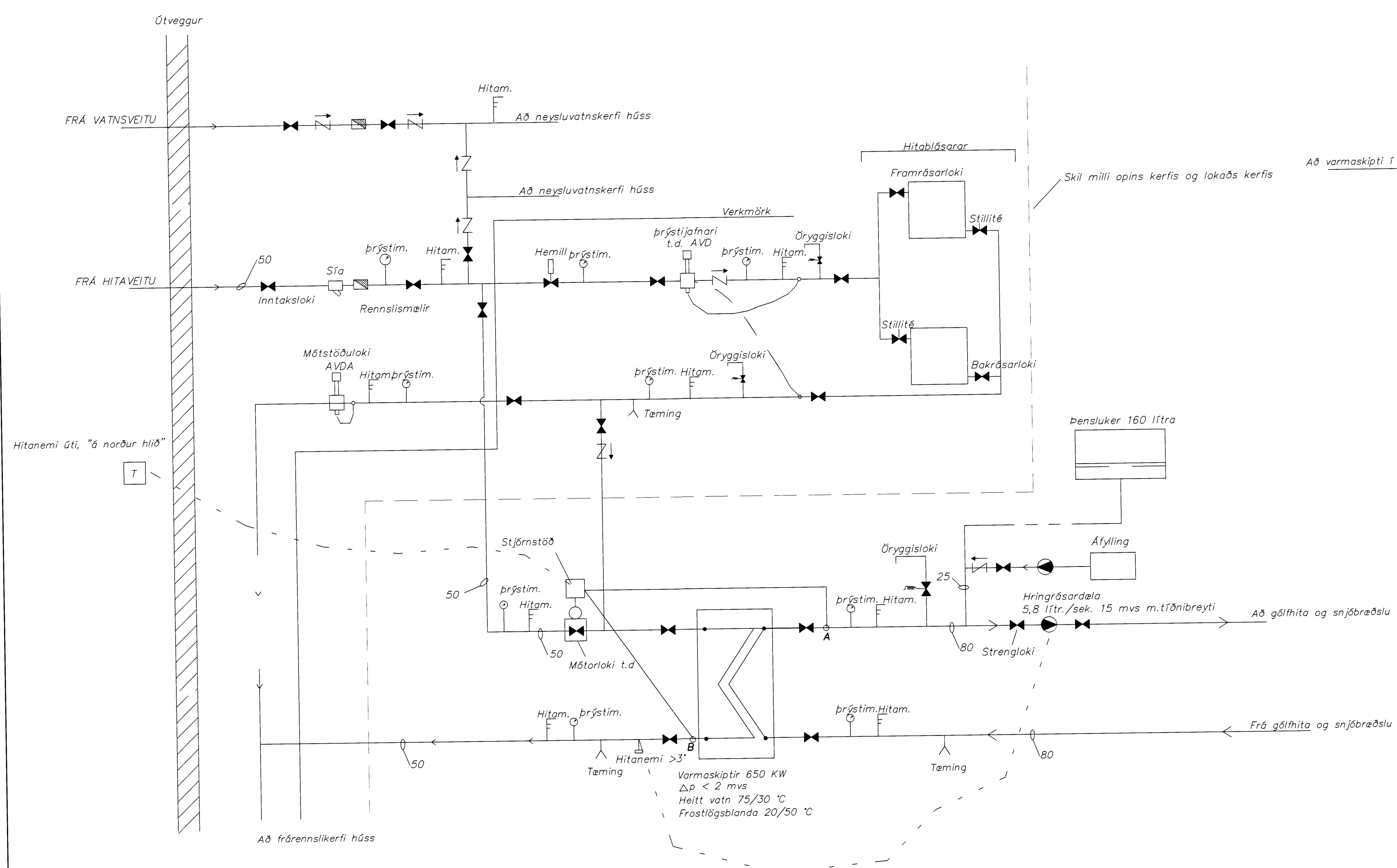
TENGIMYND HITAVEITU Í INNTAKSKLEFA
