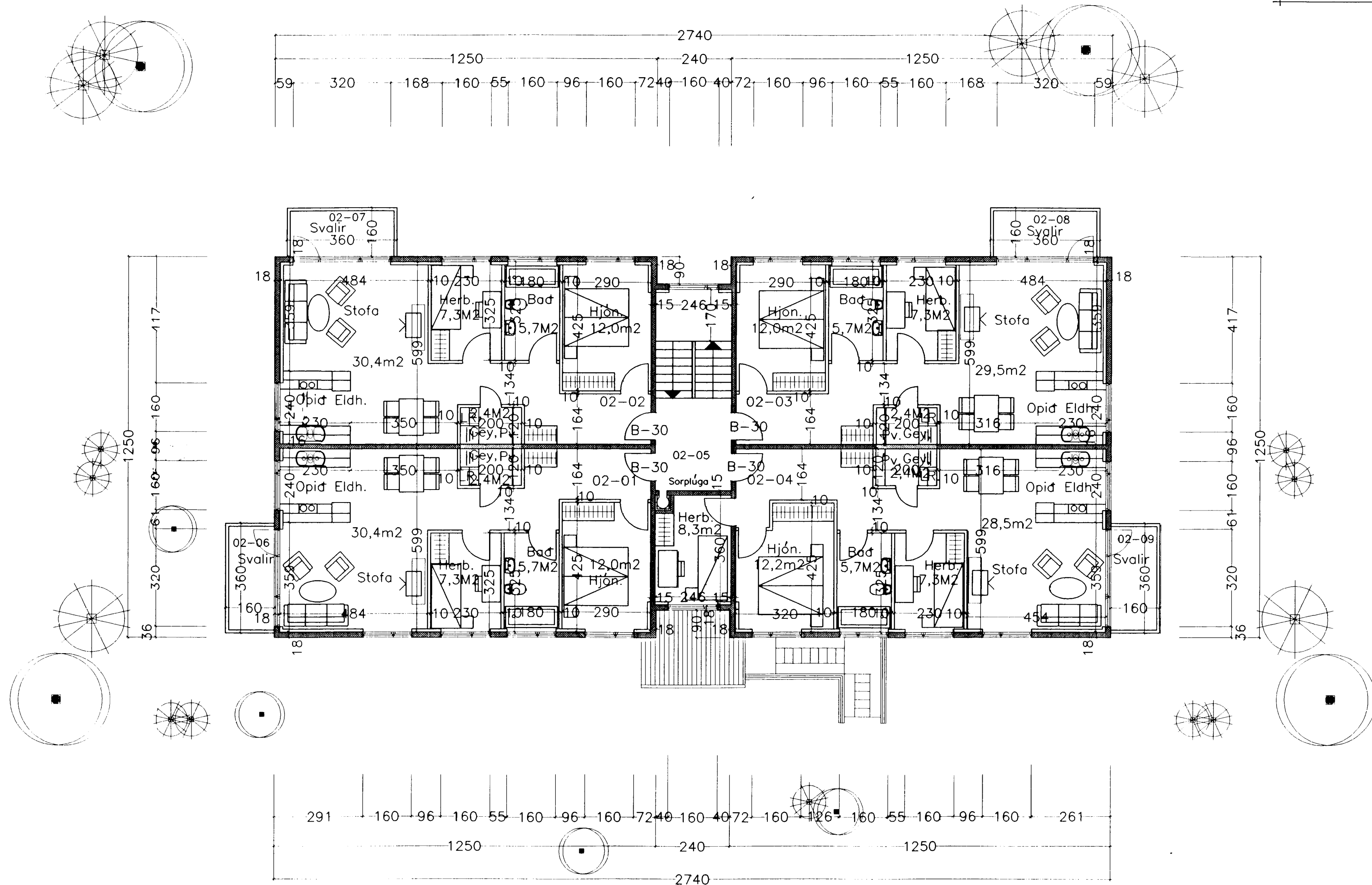
Grunnmynd 2 hæðar.
