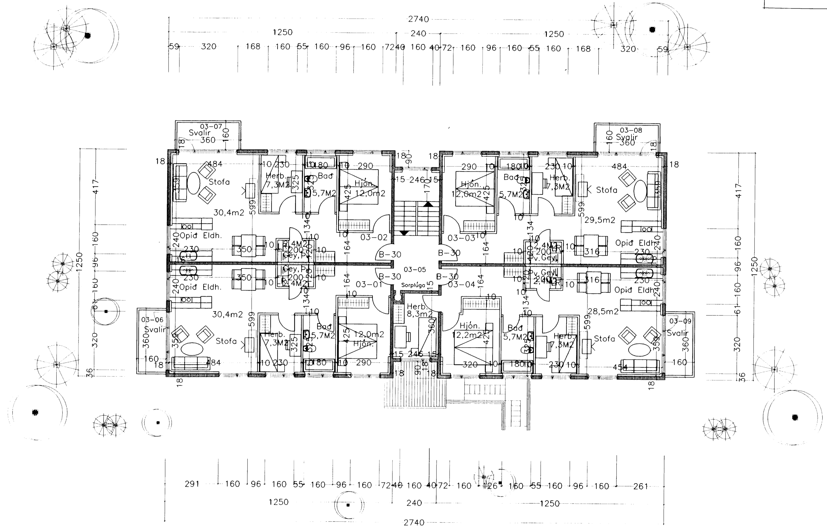
Grunnmynd 3 hæðar.
