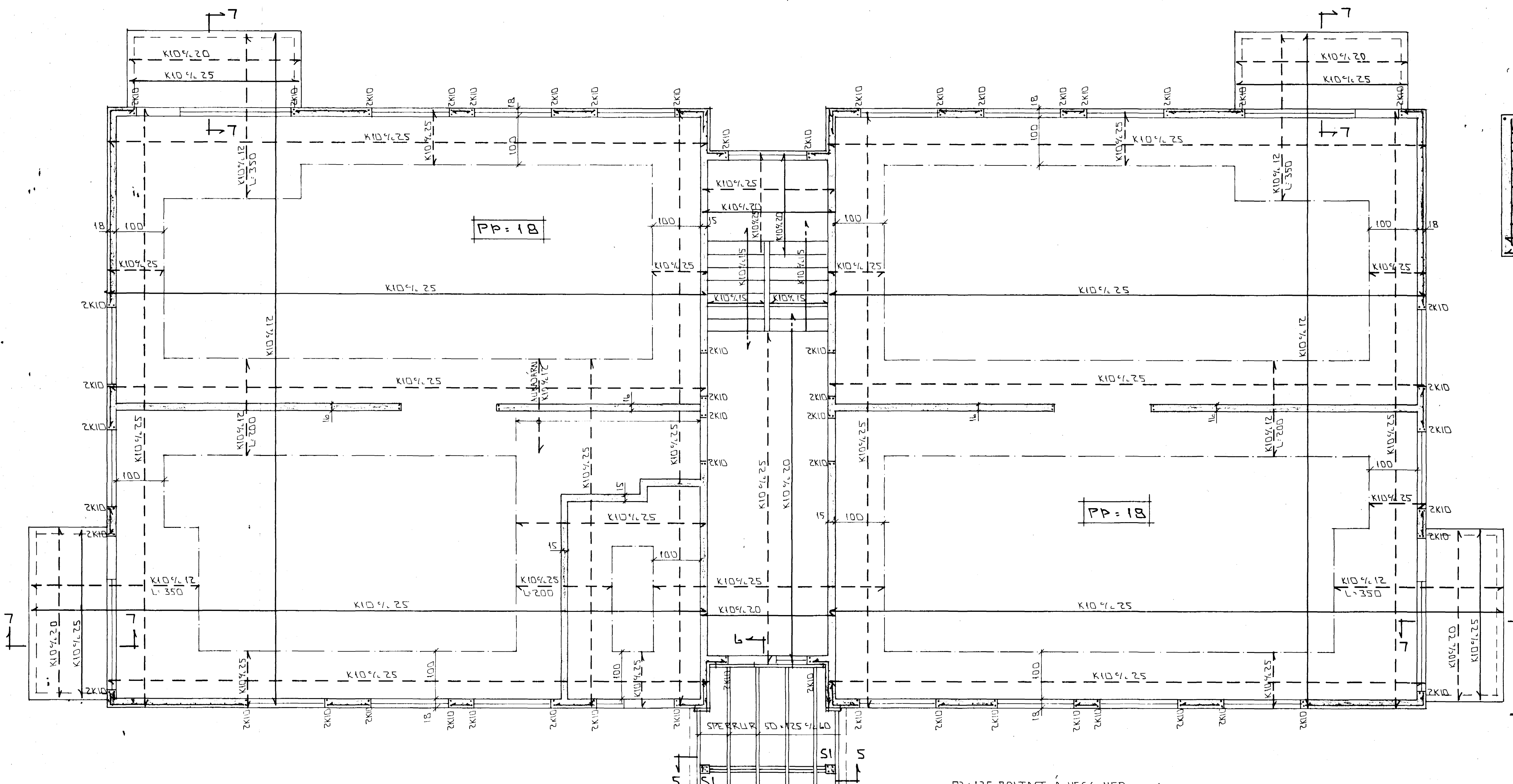
GRUNNMÝND * 1:50
