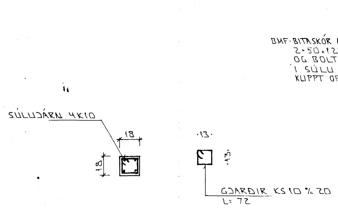
SÚLA S1 * 1:20
