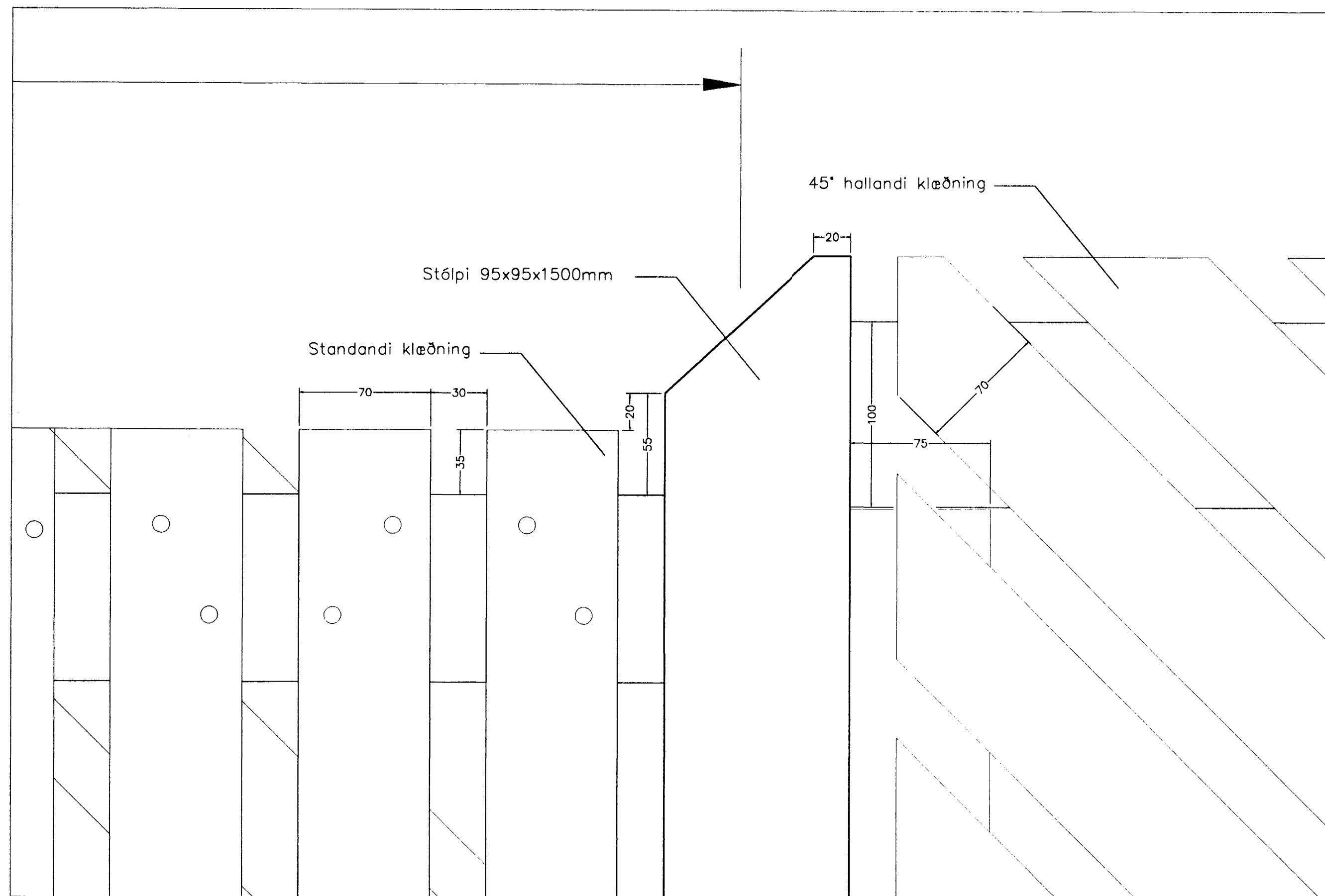
Frágangur efri hluta stólpa mkv. 1:2
