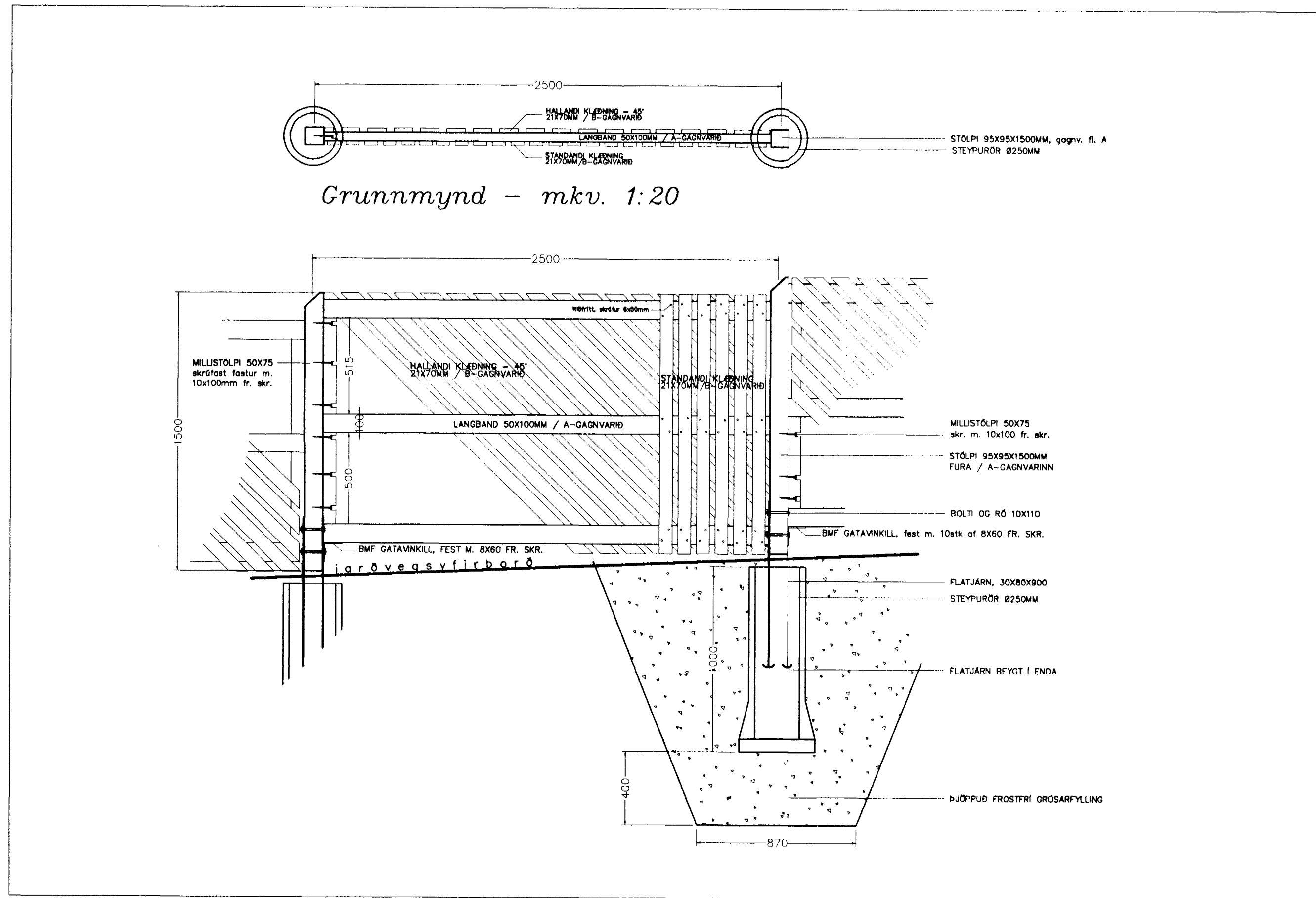
Útlit og lengdarsnið - mkv. 1:20
