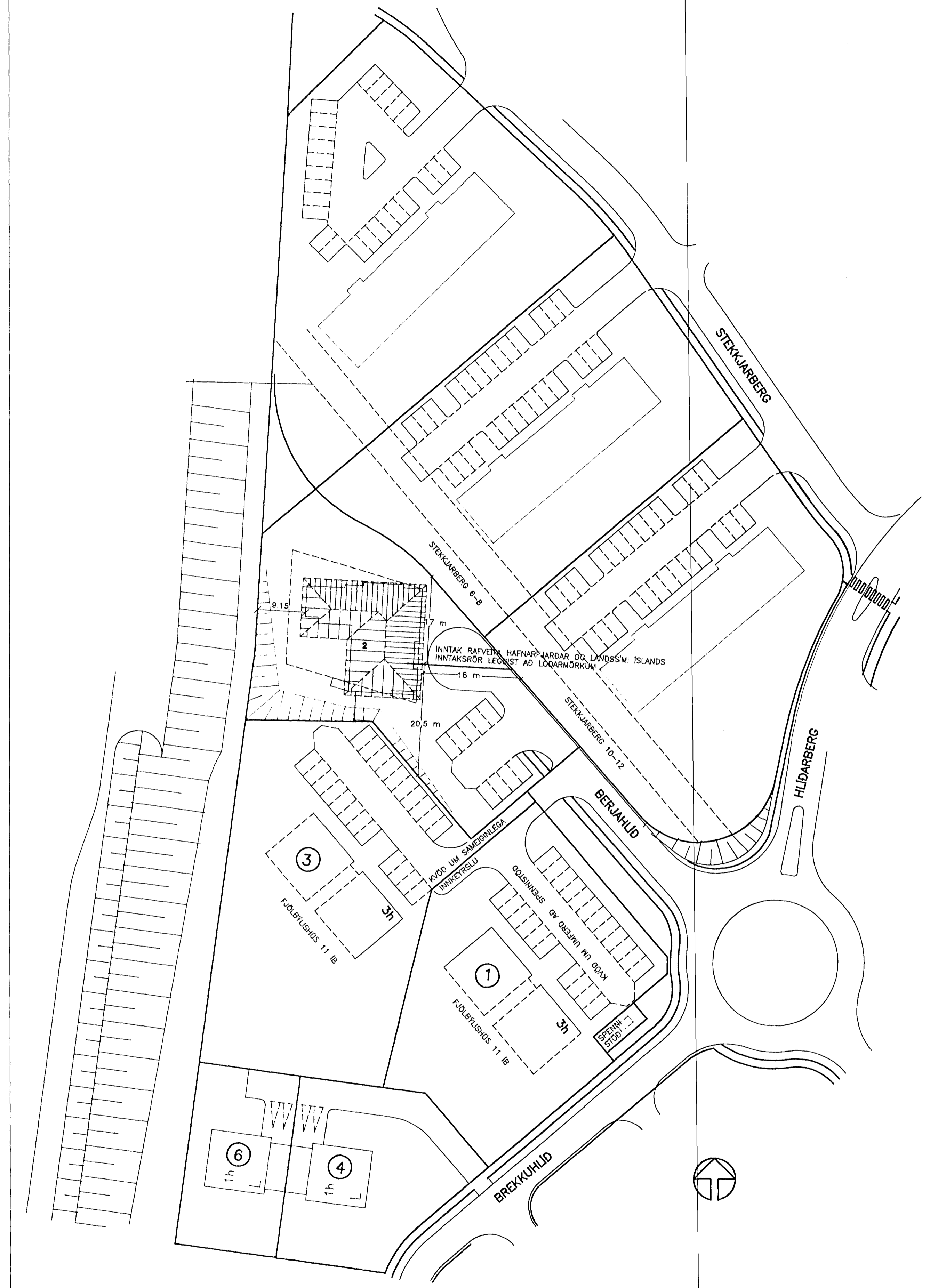
AFSTÖDUMYND MKV. 1:500
