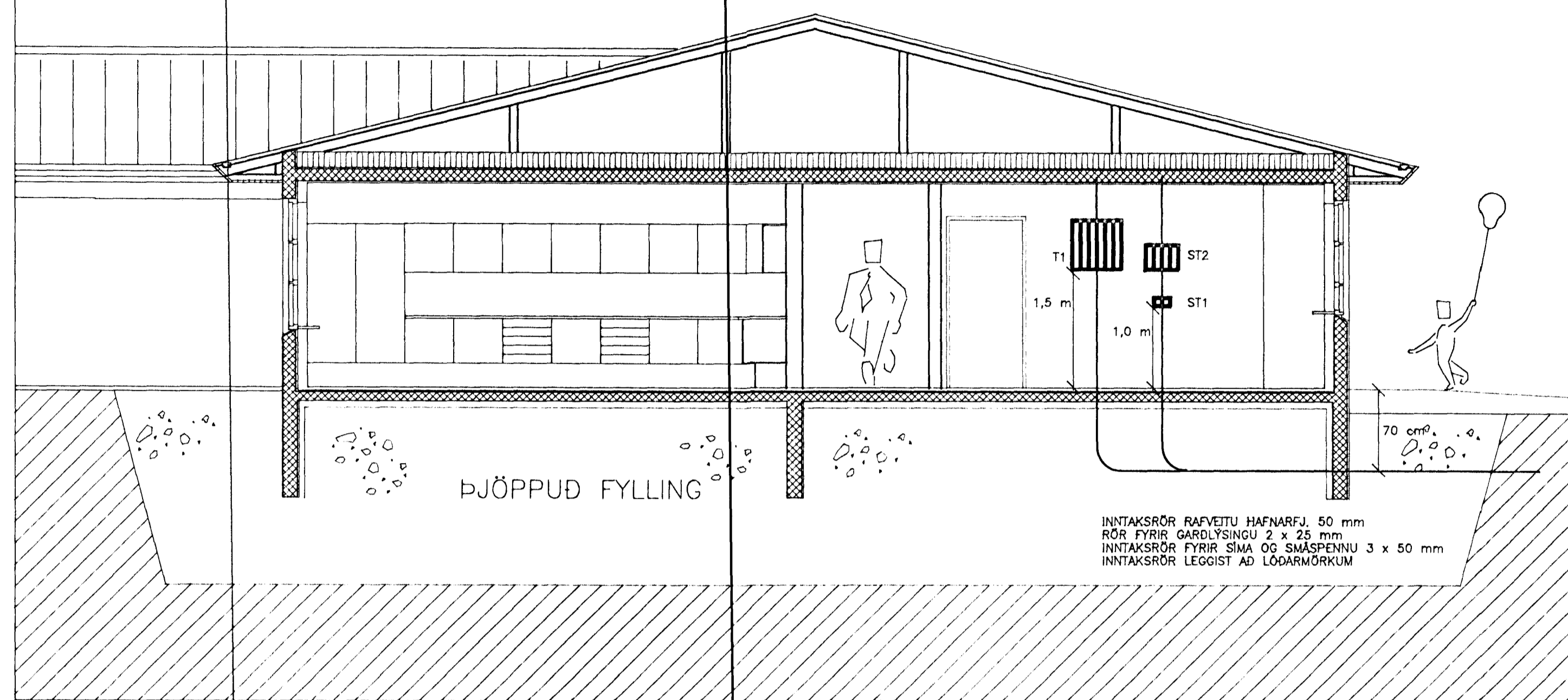
SNID MKV. 1:50
